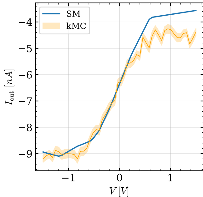
Sigmoid
