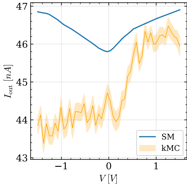
Parabola
