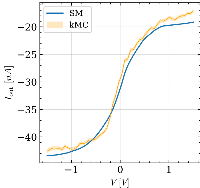
Sigmoid
