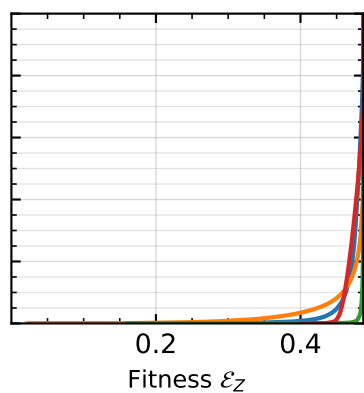
Sine
