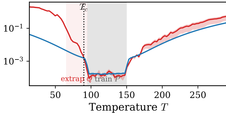
(b) ARPES
