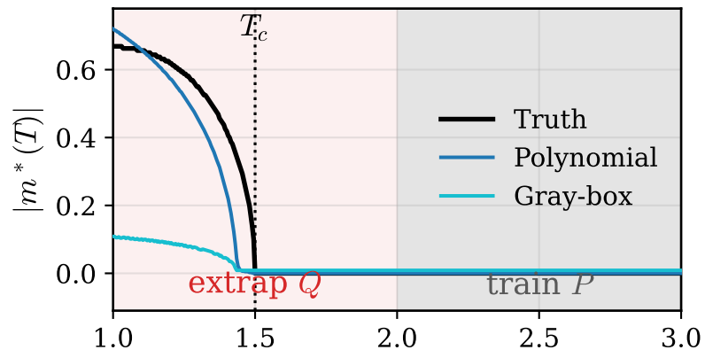
(b) Order parameter |m^*(T)|
