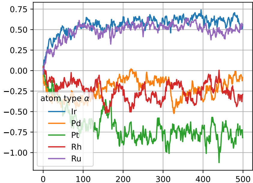
Pt- \alpha Cowley SRO parameter
