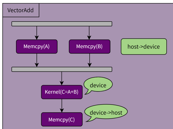
图 3.4 VectorAdd 任务图
