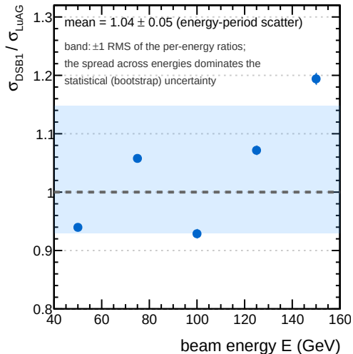
B width ratio per energy
