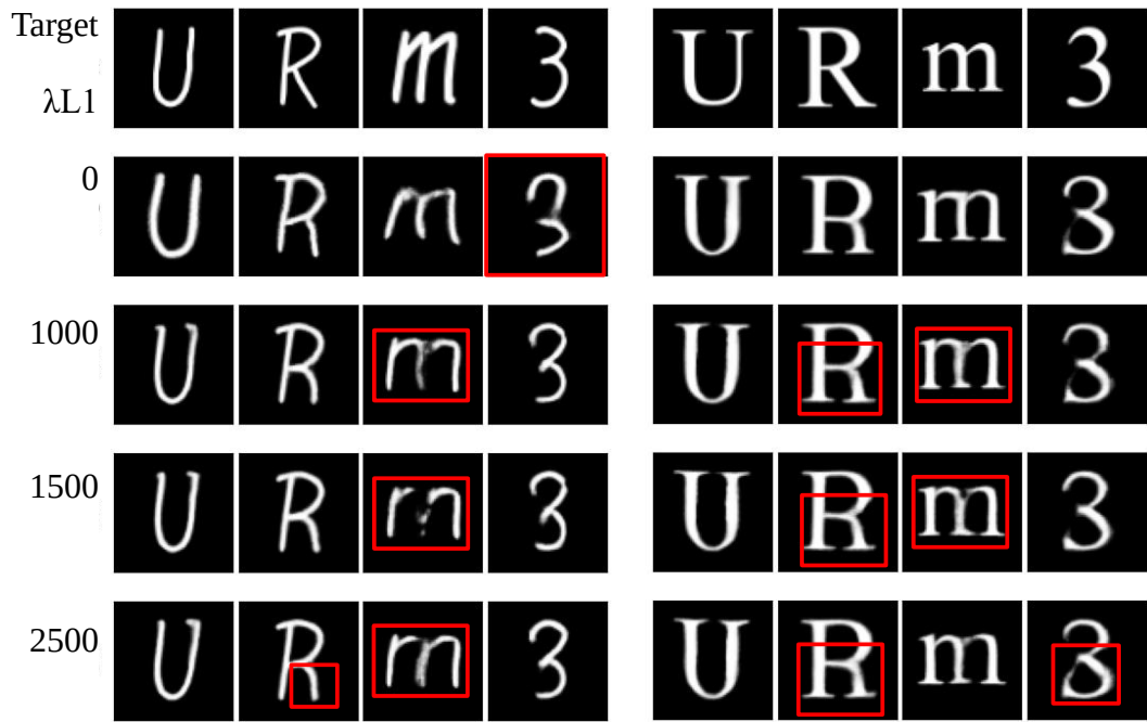
圖 25：於字體 A（左）及字體 C（右），不同的 L1 損失權重 \lambda_{L1} 對瓶頸層尺寸為 4×4 的模型生成效果之影響（紅框：較差之處）
