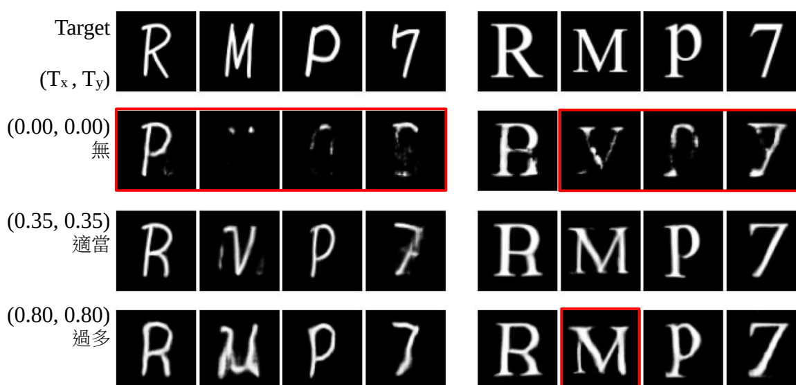
圖 11：不同平移變換參數 (T_x, T_y) 對生成結果之影响（紅框：較差之處）
