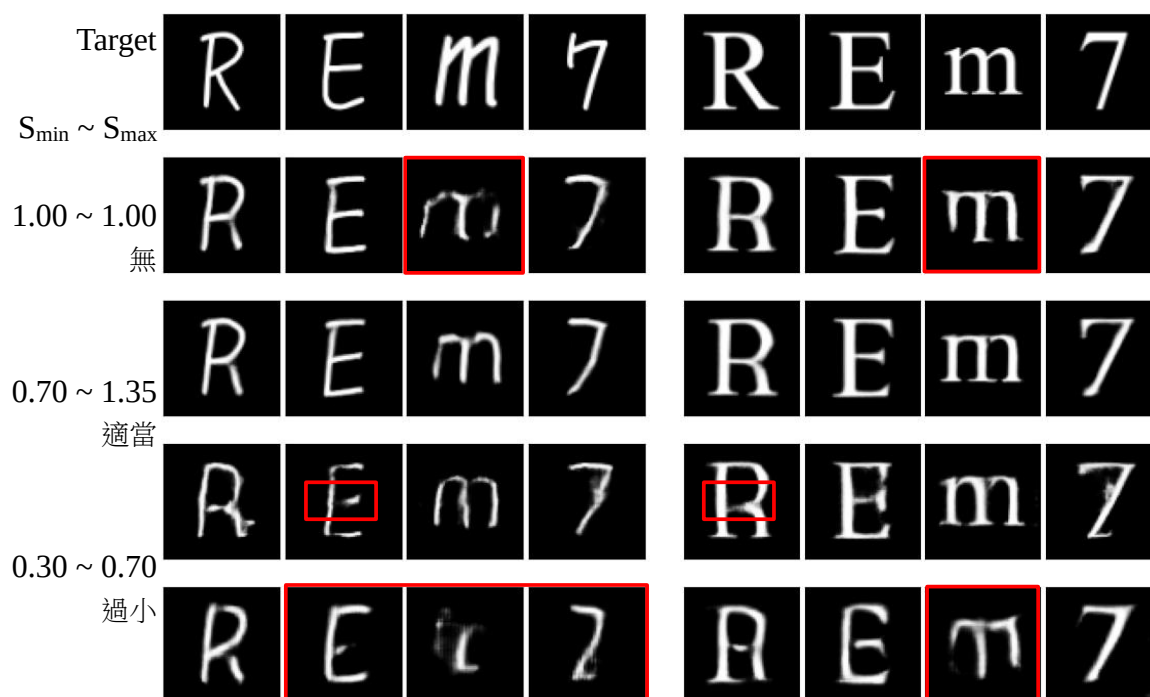
圖 10：不同縮放變換參數 S_{min} \sim S_{max} 對生成結果之影响（紅框：較差之處）
