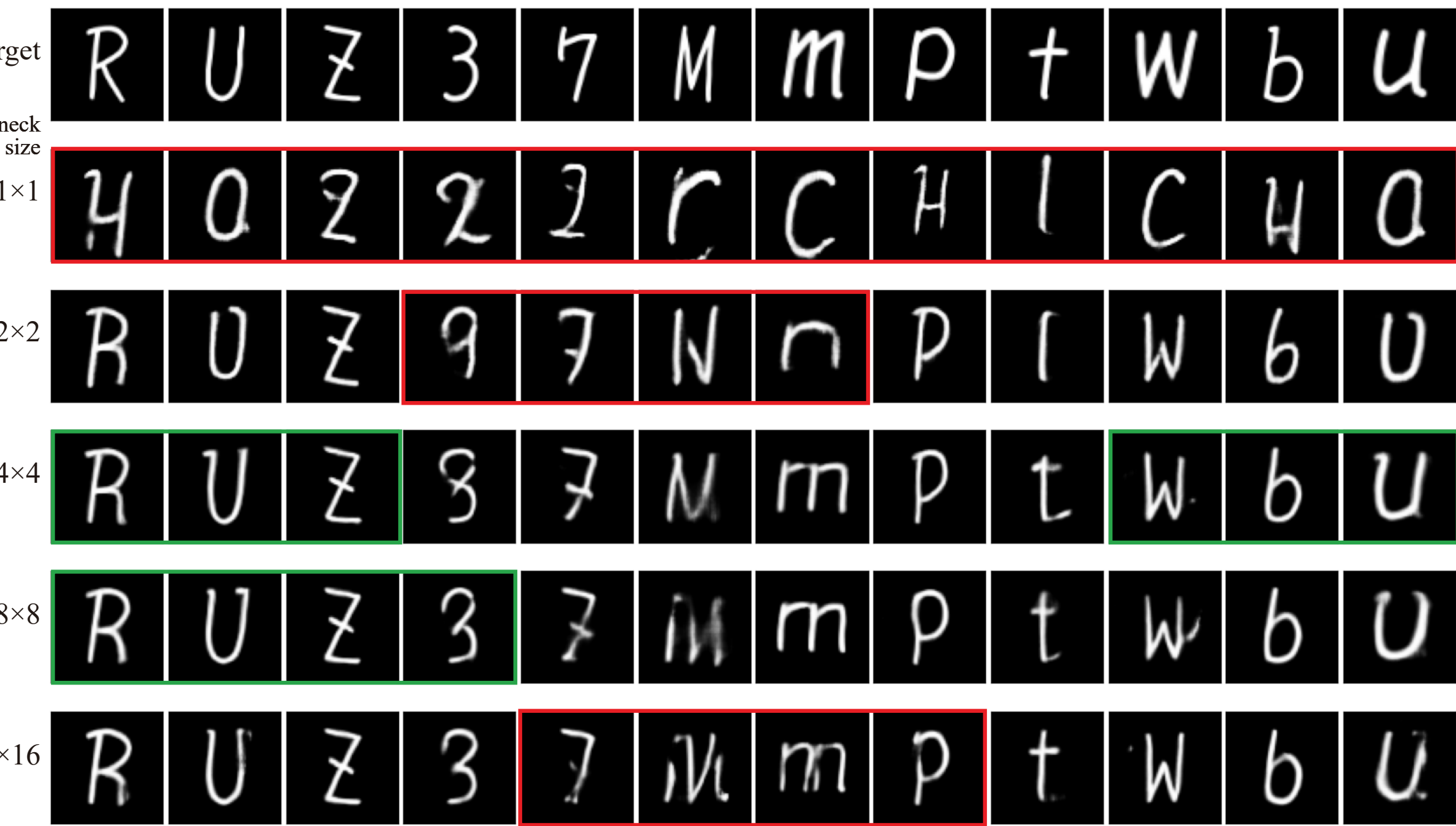
圖 12：不同瓶頸層尺寸 n=1,2,4,8,16（依序）對字體 A 的生成效果影響（第一列為目標）
