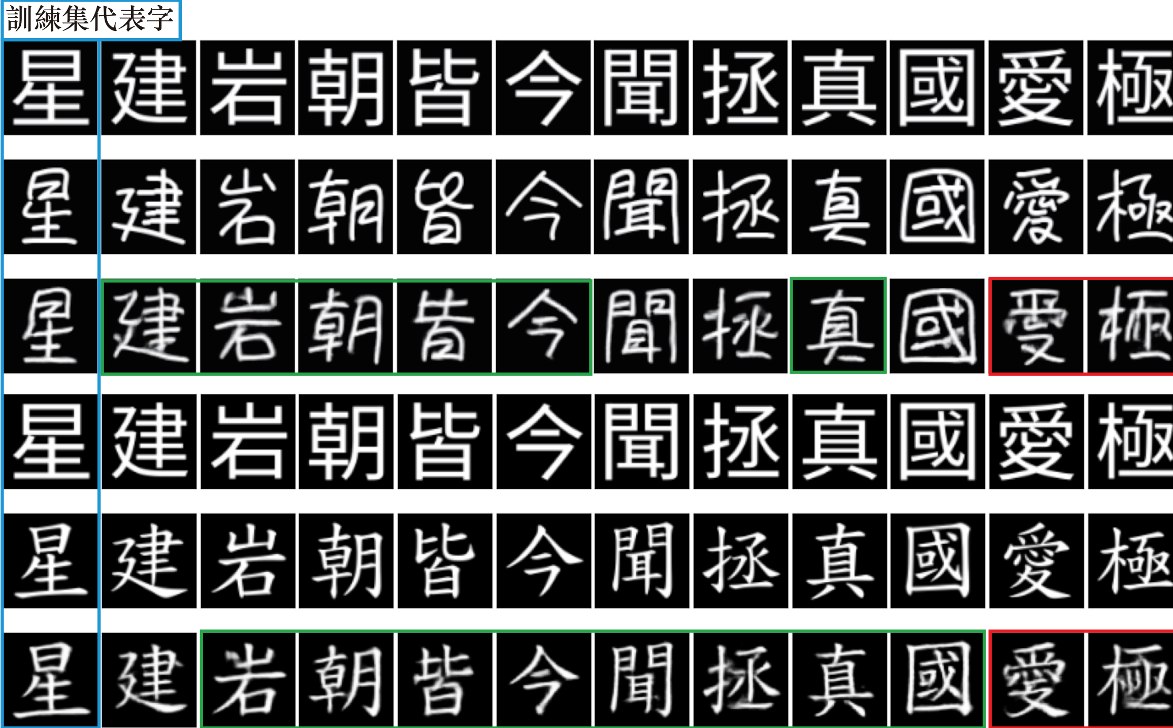
圖 20：將本研究架構應用於中文字體生成之效果成效
