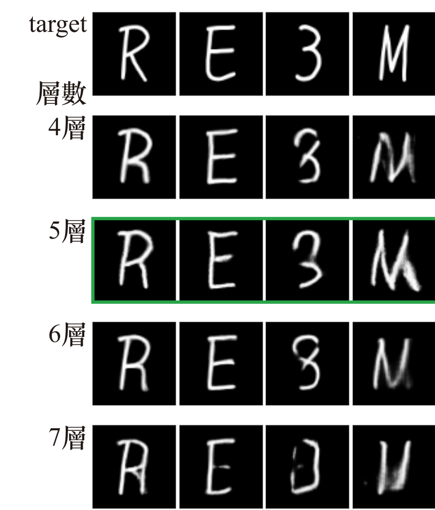
圖 17：模型層數對生成效果之影響 透過模型層數調整，排除參數量的影響（圖 21）
