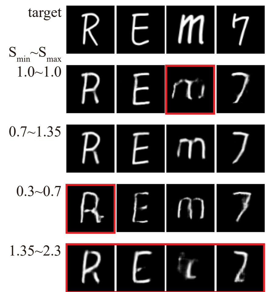
圖 8：不同縮放程度對生成結果之影響
