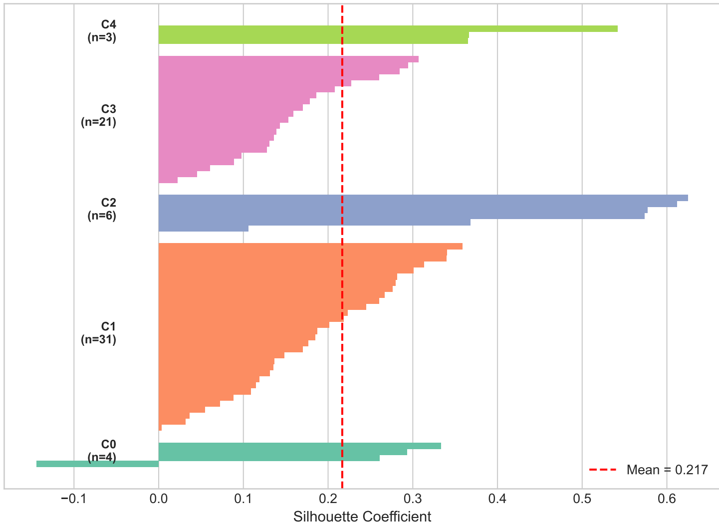
Silhouette Diagram (k=5)
