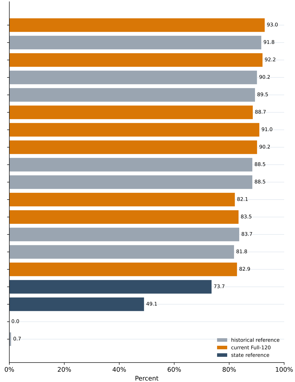
Macro-F1
