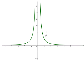
Figura 8: Gráfica de la función f(x) = 1/x^2
