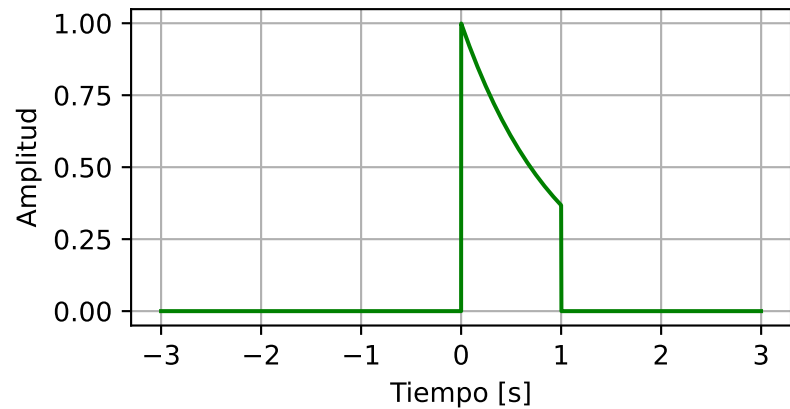
Respuesta a impulso h(t) : Exp. decreciente
