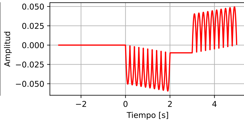
Salida y(t) = x(t) * h(t)
