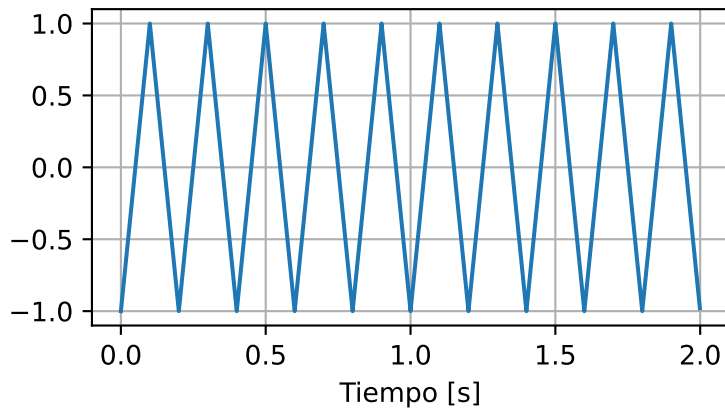
Entrada x(t) : Triangular
