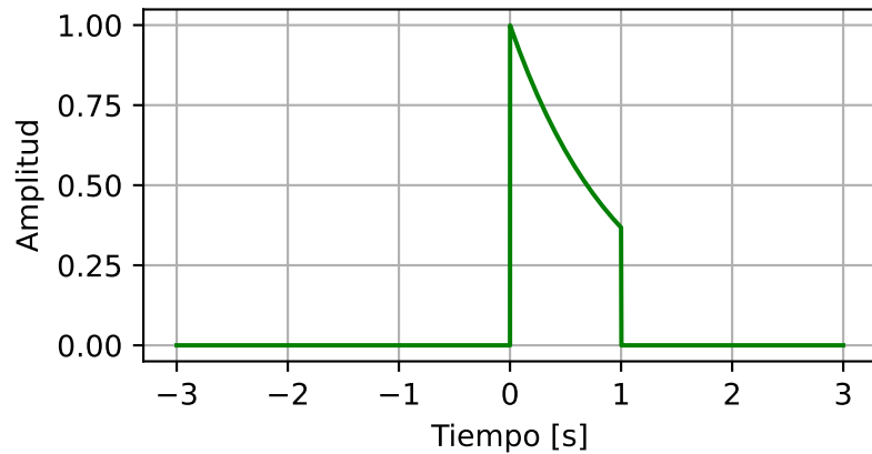
Respuesta a impulso h(t) : Exp. decreciente (original)
