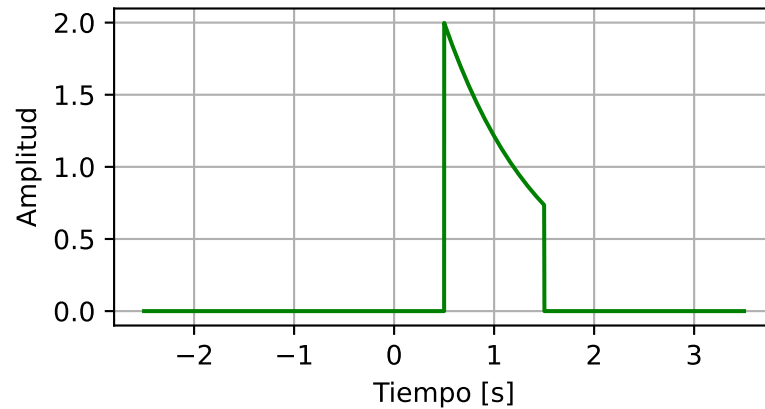
Respuesta a impulso h(t) : 2 \cdot \text{Exp. decreciente}(t - 0.5)
