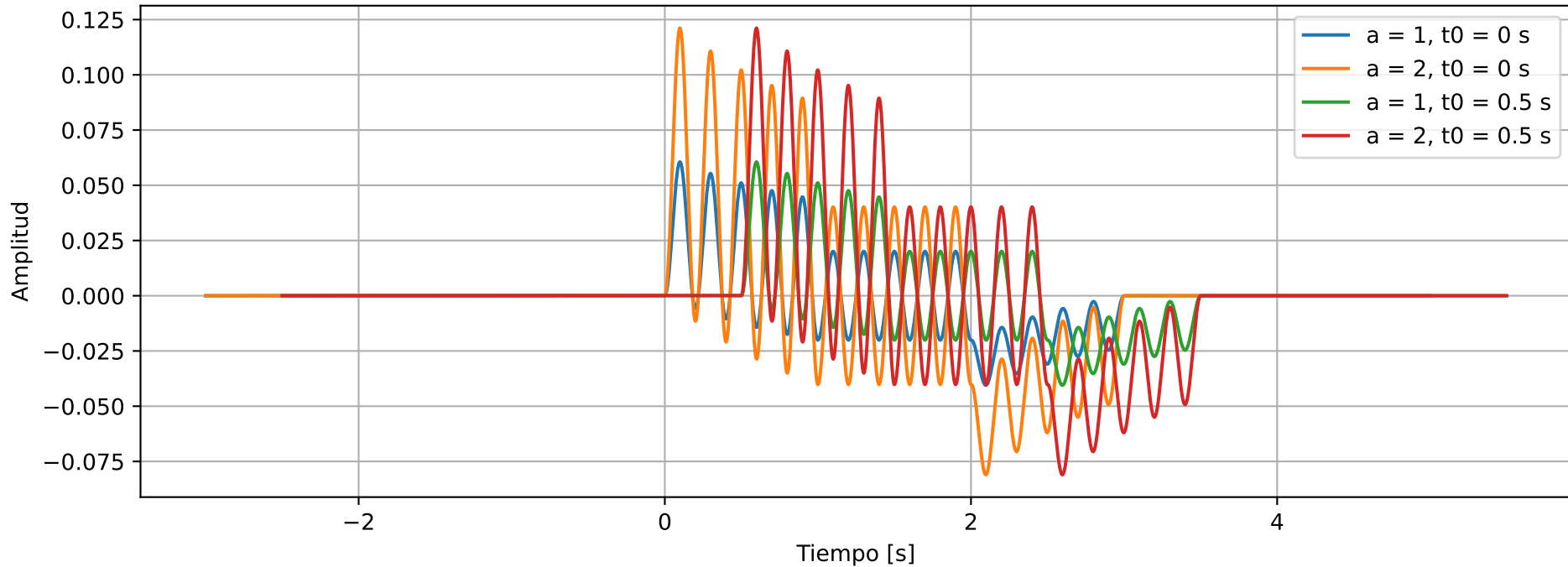
Salidas con distintos a y t_0 (entrada senoidal)
