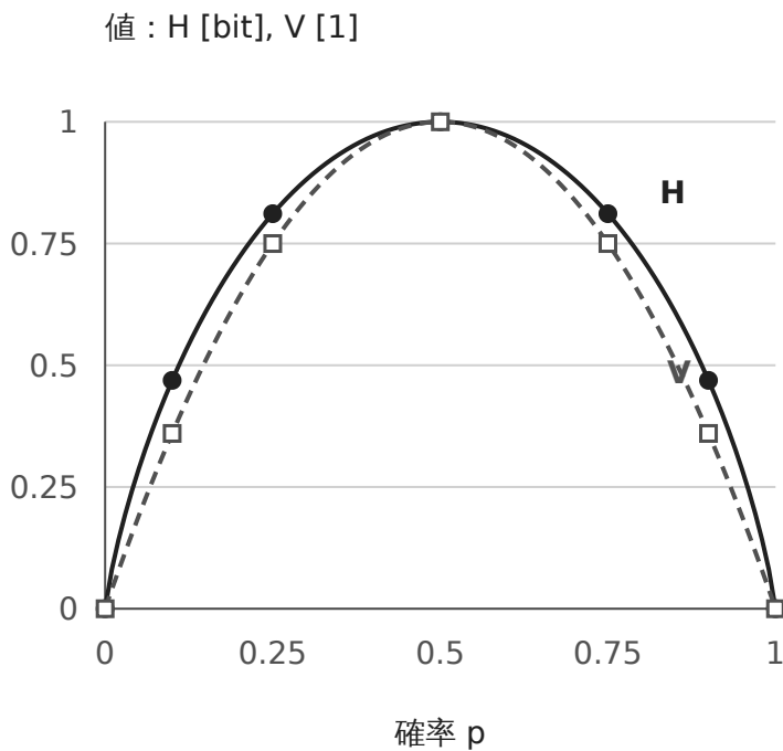
図2 ビット単位のエントロピー H と、無次元の正規化分散 V 。どちらも p = 1/2 で一となる。曲線の刻み幅は0.01、記号は表の確率に対応する。
