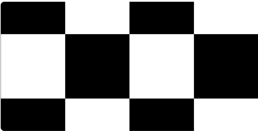
図4 確率場を二値化した画像。黒は p \geq 1/2 、白は p < 1/2 を表す。同梱したPNGの元の画素は黒と白だけである。
