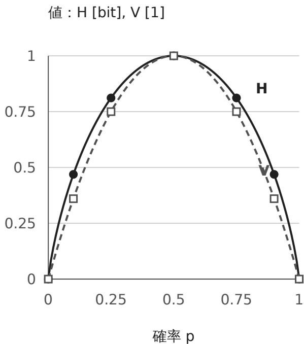
図2 ビット単位のエントロピー H と、無次元の正規化分散 V 。どちらも p = 1/2 で一となる。曲線の刻み幅は0.01、記号は表の確率に対応する。
