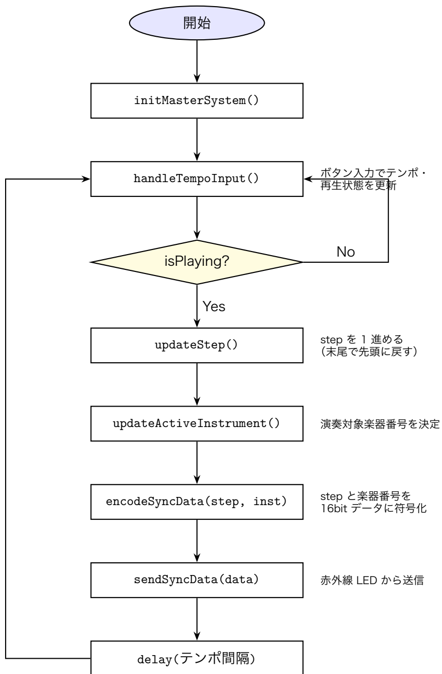
図 3.2 親機 Arduino の処理フロー
