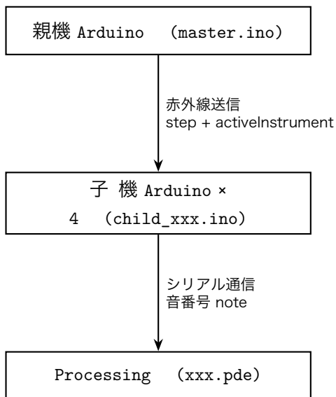
図 3.5 コンポーネント間のデータフロー
