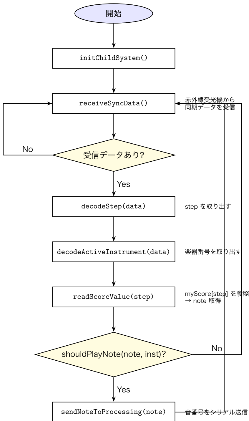
図 3.3 子機 Arduino の処理フロー（各楽器共通）
