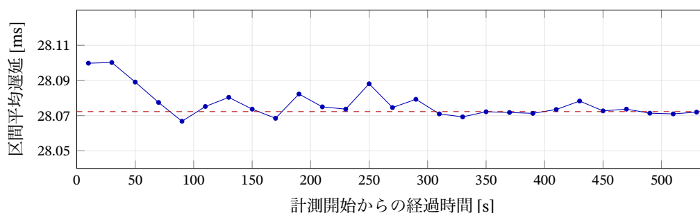
図11 片道遅延の20s区間平均の推移（破線は全体平均 28.072\text{ ms} ）
