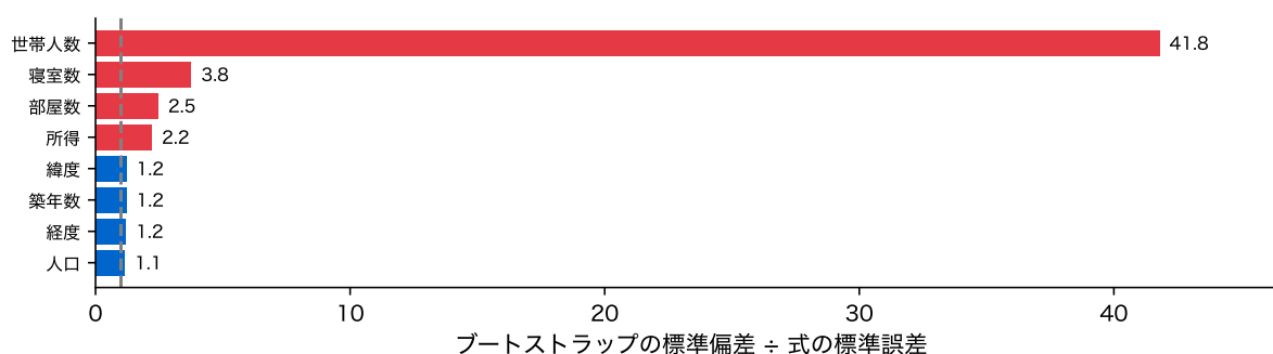
図 20: 地区を復元抽出して 1000 回当てはめ直したときの係数の標準偏差を、式の標準誤差で割った比。破線は 1 (式どおり)
