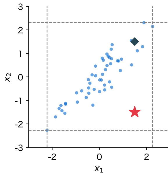
図 13: 相関 0.9 の 2 列(人工データ、50 行)。破線は各列の最小値と最大値。★はどちらの列も範囲の中だが雲の外の点、◆は原点から同じ遠さで雲に沿った点
