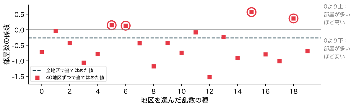
図 2: 20,640 地区から 40 地区を選んで当てはめた部屋数の係数(標準偏差 1 つぶんあたり、20 回)。破線は全地区で当てはめた値、○は符号が逆になった回
