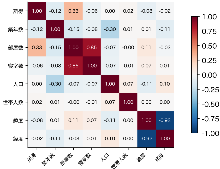
図 16: カリフォルニア住宅データの 8 列の相関行列
