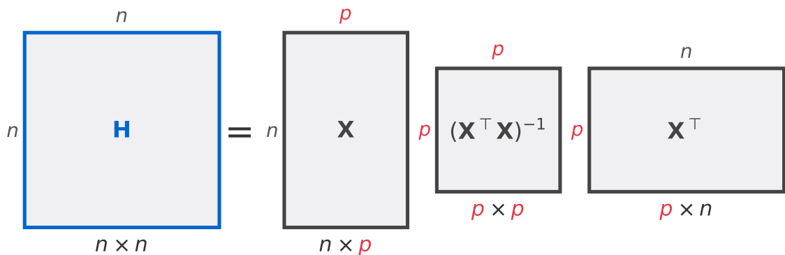
図 8: 射影行列 \mathbf{H} = \mathbf{X}(\mathbf{X}^\top \mathbf{X})^{-1} \mathbf{X}^\top の大きさ(概念図)。箱の縦は行の数、横は列の数。赤は掛け算でそろった次元
