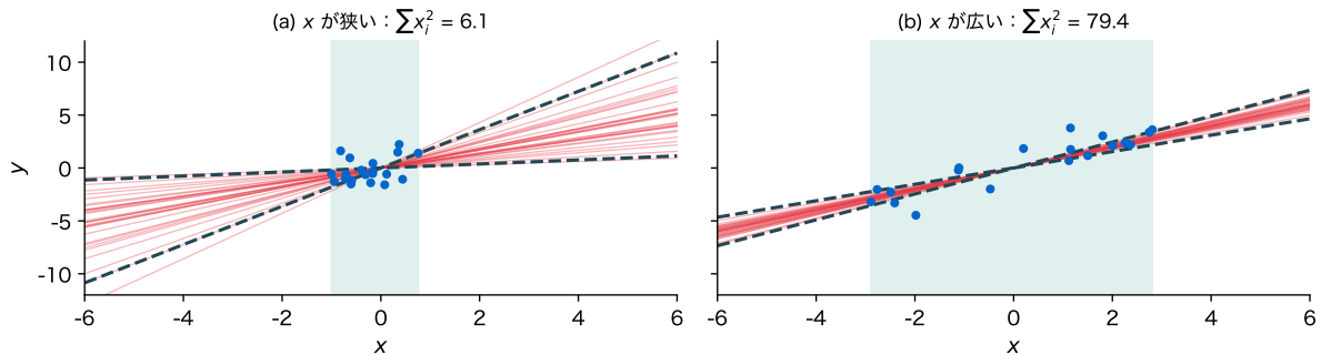
図 4: 人工データで、 x を固定したまま y を 30 回取り直して引いた原点を通る直線(赤)。(a) x が狭い範囲、(b) 広い範囲。青は 1 回ぶんの点、緑はデータのある範囲、破線は予測の \pm 2 標準偏差(後述)
