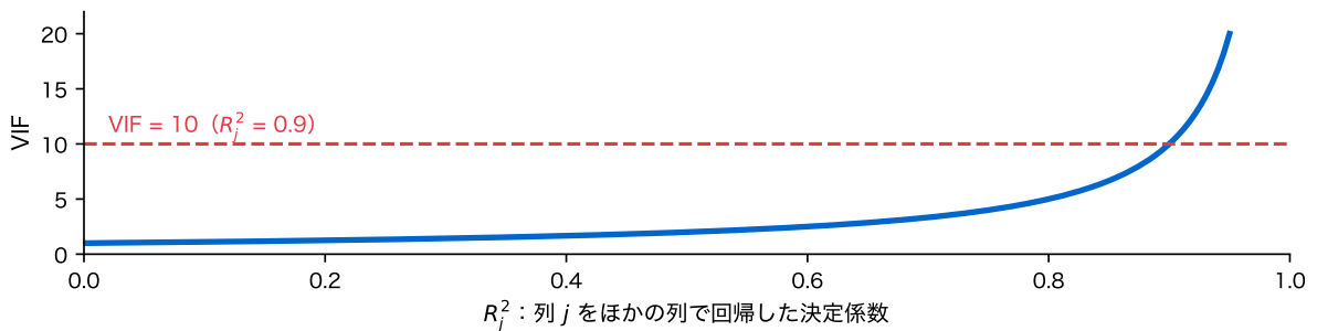
図 7: 分散拡大係数 \text{VIF}_j = 1/(1-R_j^2) と、目安とされる \text{VIF} = 10 (赤の破線)
