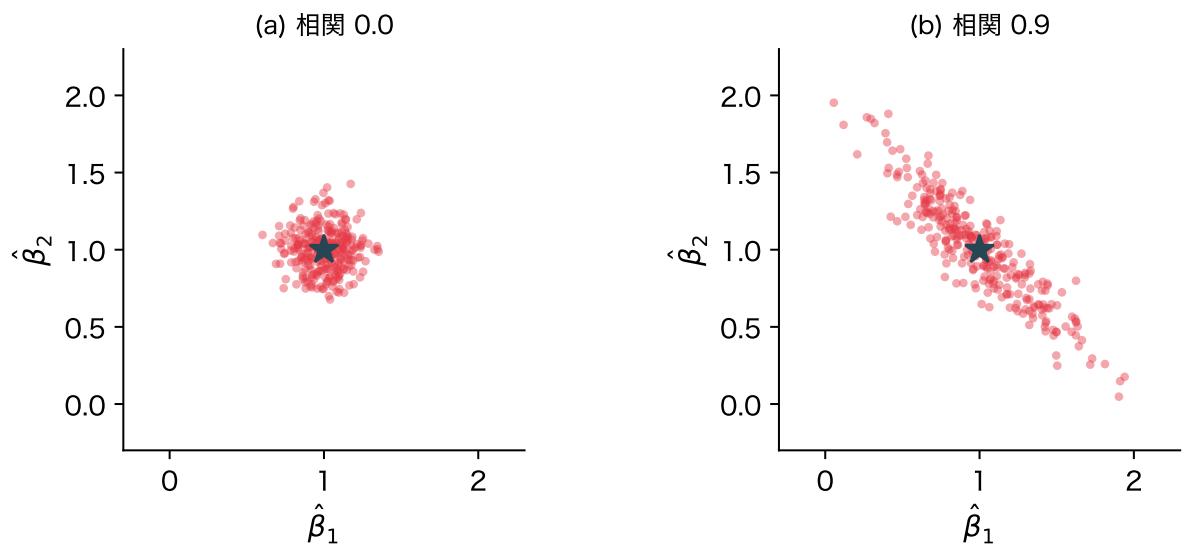
図 6: 人工データで y を 300 回取り直したときの係数の推定値。★は真の値。(a) 2 列の相関が 0、(b) 0.9
