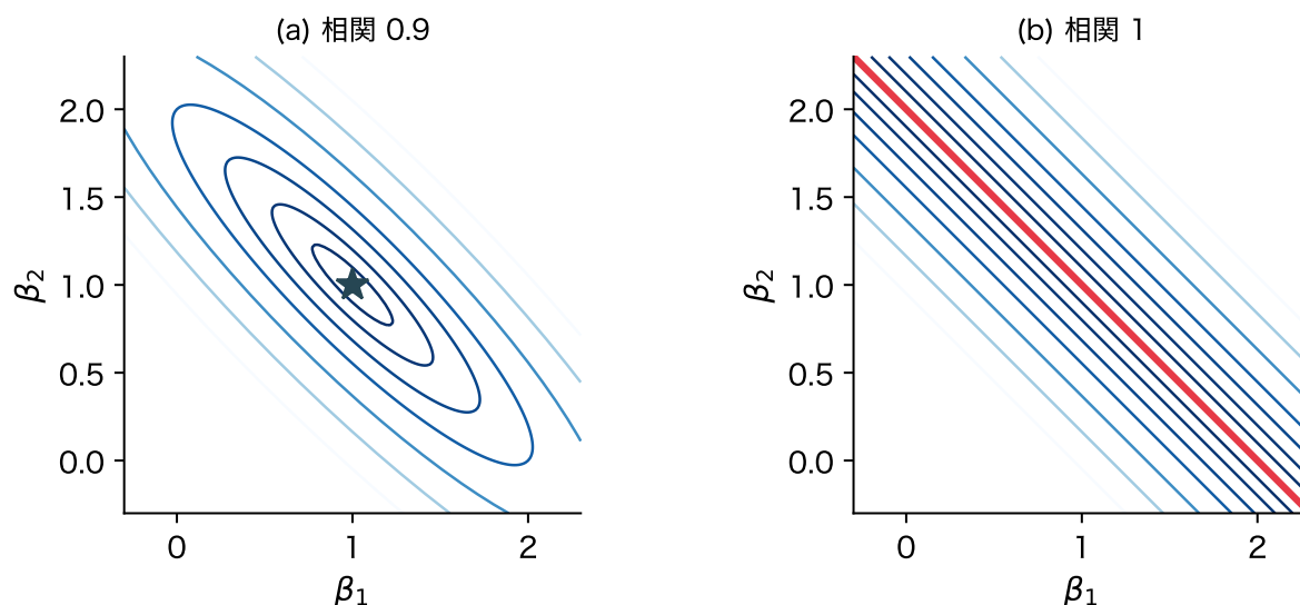
図 14: 2 列の場合の目的関数の等高線(人工データ)。(a) 相関 0.9 では底が 1 点(★)、(b) 相関 1 では底が直線(赤)になり、解が無数にある
