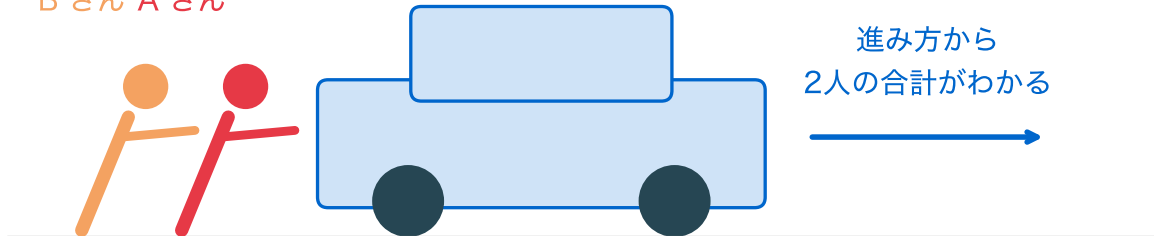
図 5: 共線性のたとえ(概念図)。いつも 2 人で押す車では、進み方から 2 人の力の合計はわかるが、内訳はわからない
