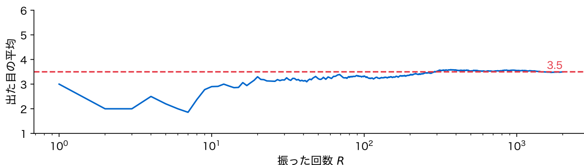
図 3: サイコロを振った回数と、それまでに出了目の平均(人工データ、2000 回)。横軸は対数。赤の破線は期待値 3.5
