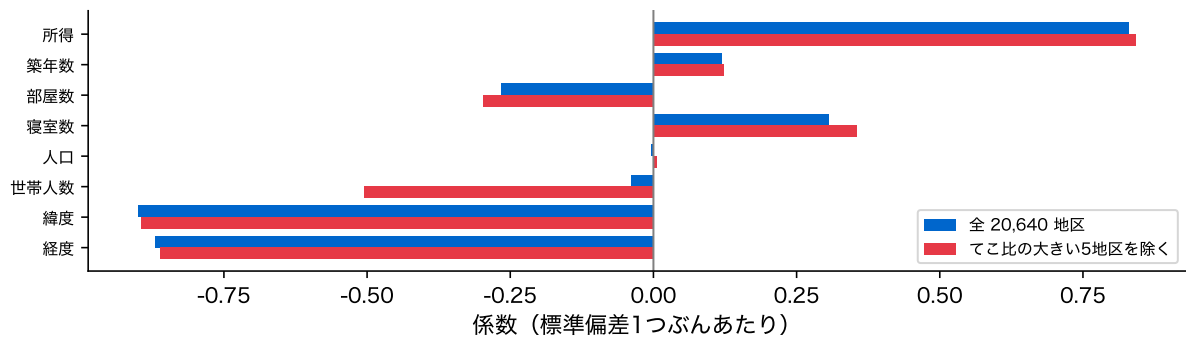
図 22: 全地区で当てはめた係数(青)と、てこ比の大きい 5 地区を除いて当てはめた係数(赤)。標準偏差 1 つぶんあたり
