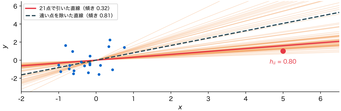
図 11: てこ比の大きい 1 点(人工データ)。青の 20 点に x = 5 の赤の点を足した。赤の実線は 21 点で、黒の破線は赤の点を除いて引いた直線。橙は 21 行を復元抽出して引き直した直線(80 回ぶん)
