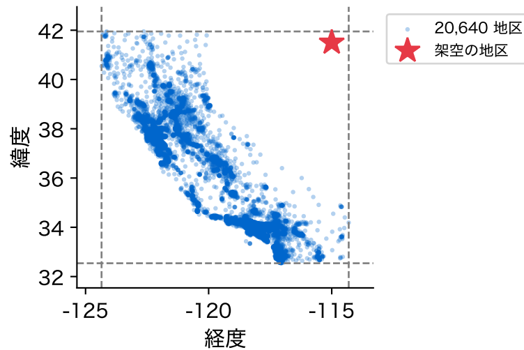
図 23: 地区の緯度と経度と、架空の地区(★)。破線は緯度・経度それぞれの最小値と最大値
