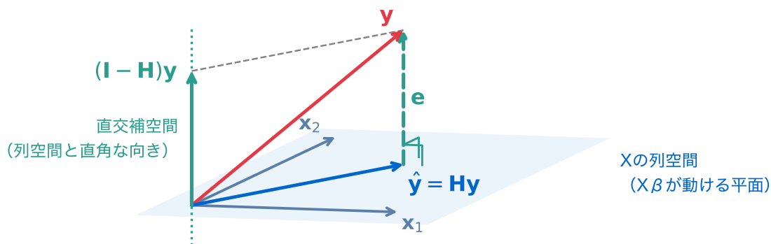
図 9: 観測 \mathbf{y} を、 \mathbf{X} の列空間への影 \hat{\mathbf{y}} = \mathbf{H}\mathbf{y} と、直交補空間(点線)への影 (\mathbf{I} - \mathbf{H})\mathbf{y} = \mathbf{e} に分ける(概念図)。残差 \mathbf{e} は平面に垂直で、どの列とも直交する
