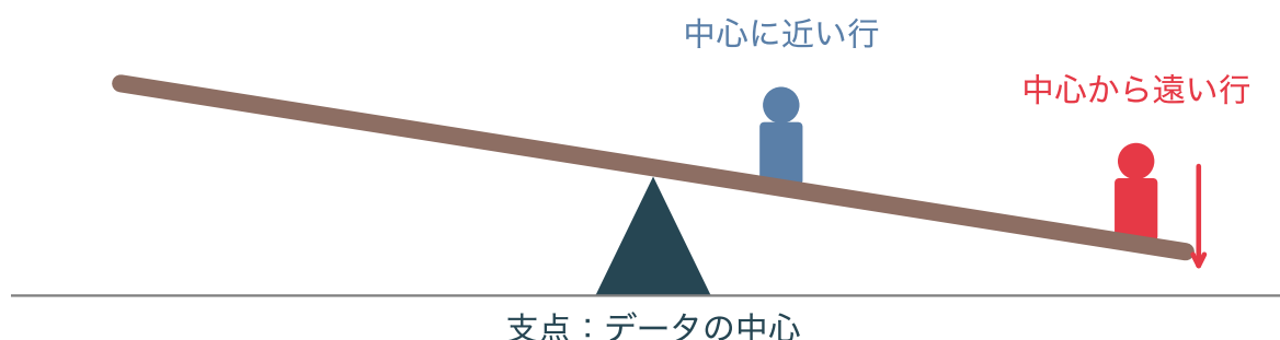
図 10: てこ比のたとえ(概念図)。直線はデータを中心を支点に回る板で、中心から遠い行ほど板を大きく傾ける
