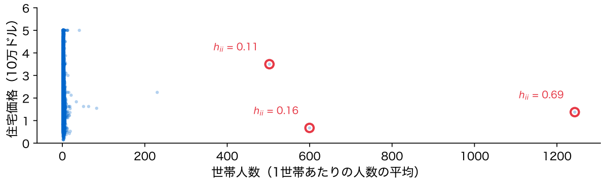
図 21: 世帯人数と住宅価格。赤丸は世帯人数の大きい 3 地区で、数字はそのてこ比
