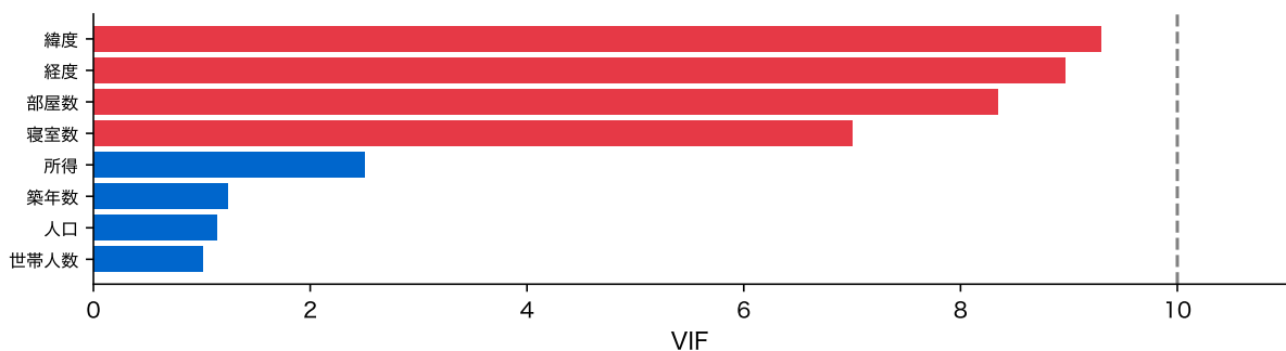
図 19: カリフォルニア住宅データの 8 列の VIF。赤は 5 以上の列、破線は目安とされる VIF = 10
