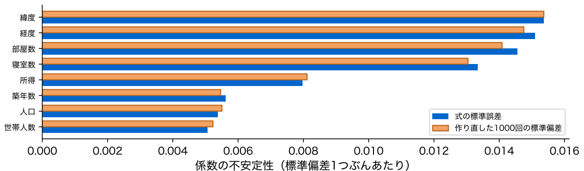
図 17: 係数の不安定性。式 \hat{\sigma}^2(\mathbf{X}^\top \mathbf{X})^{-1} による標準誤差(青)と、 \mathbf{X} を固定して目的変数を 1000 回作り直したときの標準偏差(橙)。標準偏差 1 つぶんあたりに直してある
