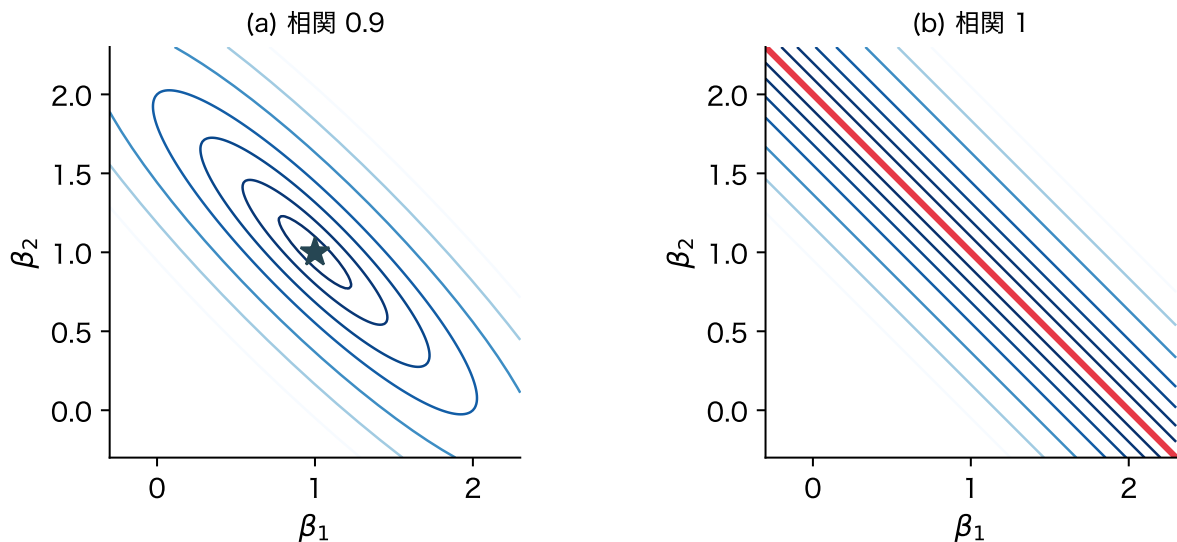
図 10: 2 列の場合の目的関数の等高線(人工データ)。(a) 相関 0.9 では底が 1 点(★)、(b) 相関 1 では底が直線(赤)になり、解が無数にある
