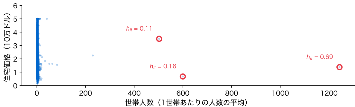
図 16: 世帯人数と住宅価格。赤丸は世帯人数の大きい 3 地区で、数字はそのてこ比
