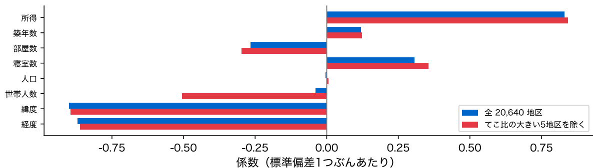
図 17: 全地区で当てはめた係数(青)と、てこ比の大きい 5 地区を除いて当てはめた係数(赤)。標準偏差 1 つぶんあたり
