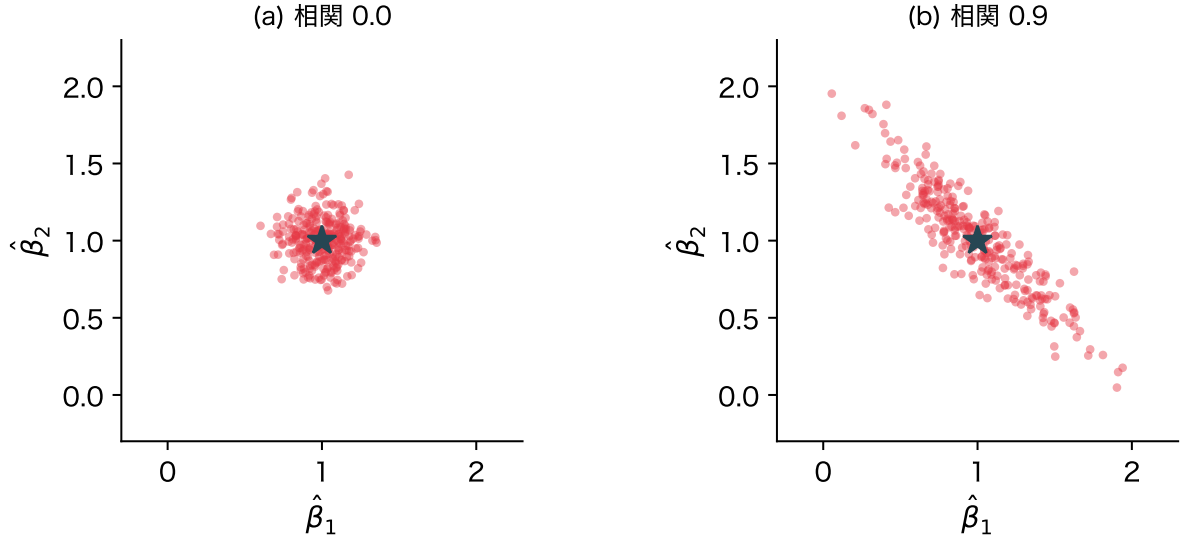
図 4: 人工データで \mathbf{y} を 300 回取り直したときの係数の推定値。★は真の値。(a) 2 列の相関が 0、(b) 0.9
