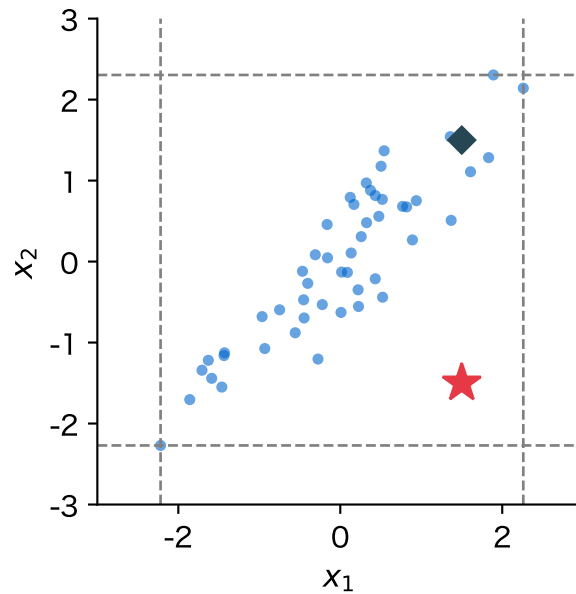
図 9: 相関 0.9 の 2 列(人工データ、50 行)。破線は各列の最小値と最大値。★はどちらの列も範囲の中だが雲の外点、◆は原点から同じ遠さで雲に沿った点
