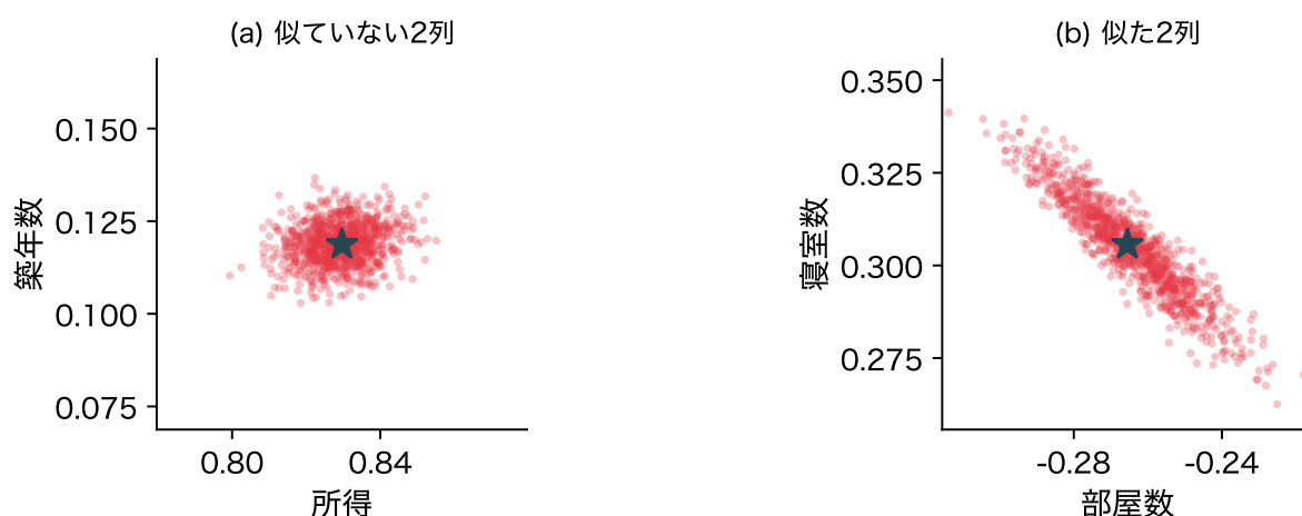
図 13: X を固定して目的変数を 1000 回作り直したときの係数(標準偏差 1 つぶんあたり)。★は全地区で当てはめた値で、2 枚とも★から \pm 0.05 の範囲を描いた。(a) 所得と築年数、(b) 部屋数と寝室数
