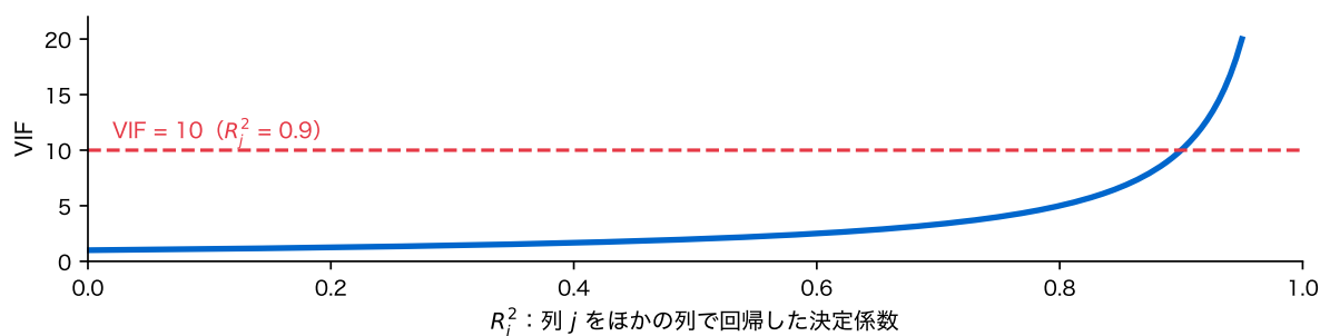
図 5: 分散拡大係数 VIF_j = 1/(1 - R_j^2) と、目安とされる VIF = 10 (赤の破線)
