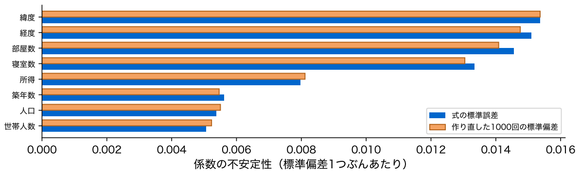
図 12: 係数の不安定性。式 \hat{\sigma}^2(\mathbf{X}^\top \mathbf{X})^{-1} による標準誤差(青)と、 \mathbf{X} を固定して目的変数を 1000 回作り直したときの標準偏差(橙)。標準偏差 1 つぶんあたりに直してある
