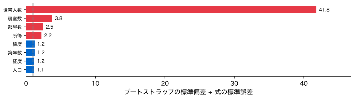
図 15: 地区を復元抽出して 1000 回当てはめ直したときの係数の標準偏差を、式の標準誤差で割った比。破線は 1 (式どおり)
