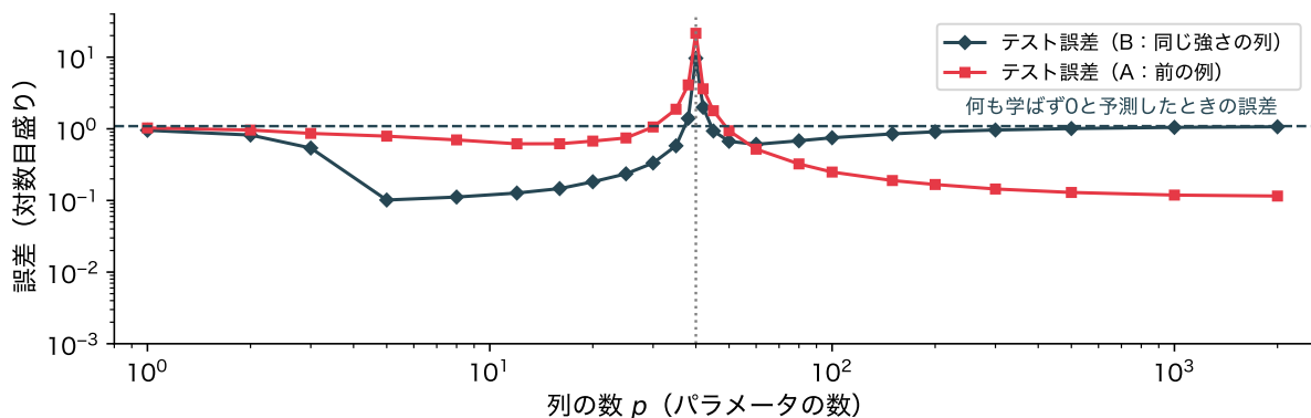
図 16: 2 つの人工データでの二重降下(テスト誤差)。A (赤)は図 15 と同じ、少数の隠れた量にノイズの乗った列。B (濃い緑)はどれも同じ強さで互いに無関係な列。破線は B で何も学ばずに 0 と予測したときの誤差。両軸とも対数目盛り
