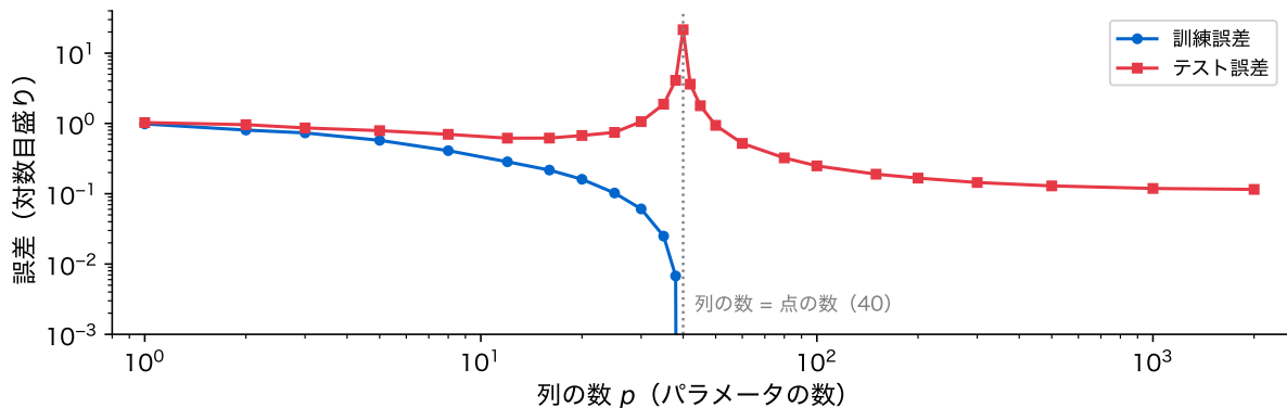
図 15: 人工データでの二重降下。訓練 40 点に、列の数 p を変えて最小二乗法を当てはめたときの訓練誤差(青)とテスト誤差(赤)。 p > 40 では係数のユークリッドノルムが最小の解を使う。 p \geq 40 の訓練誤差は 0 なので描いていない。両軸とも対数目盛り
