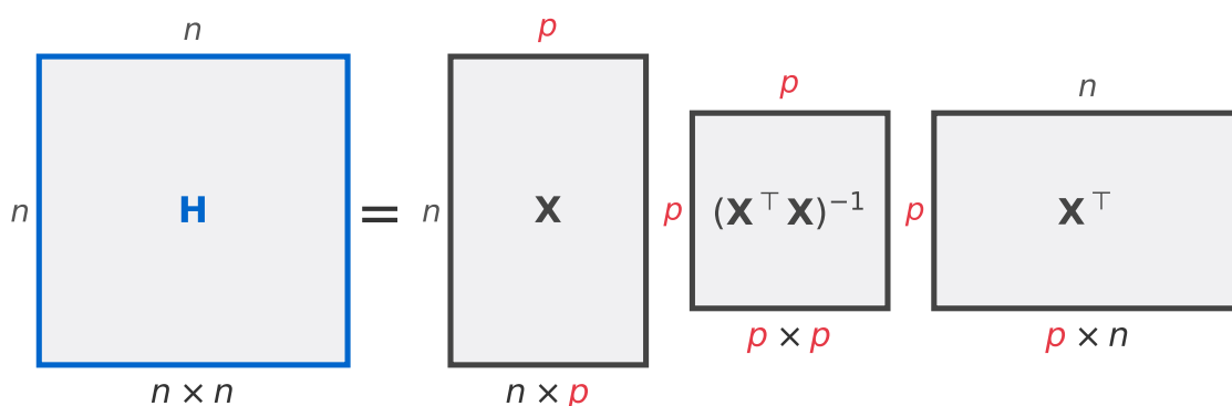
図 10: 射影行列 \mathbf{H} = \mathbf{X}(\mathbf{X}^\top \mathbf{X})^{-1} \mathbf{X}^\top の大きさ(概念図)。箱の縦は行の数、横は列の数。赤は掛け算でそろった次元
