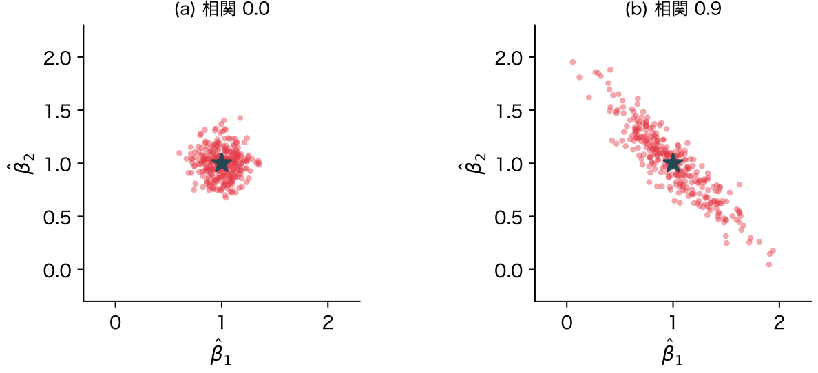
図 8: 人工データで y を 300 回取り直したときの係数の推定値。★は真の値。(a) 2 列の相関が 0、(b) 0.9
