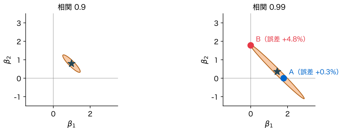
図 28: 羅生門集合(人工データ、50 行)。訓練の二乗誤差が最小(★)から 5% 以内の係数の組(橙)。(左) 相関 0.9、(右) 相関 0.99。A は列 1 だけ、B は列 2 だけを使うモデル
