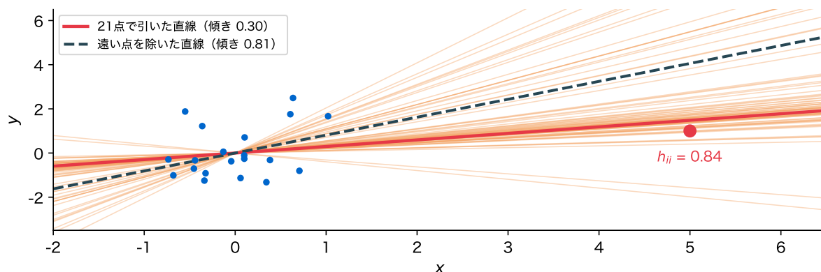
図 14: てこ比の大きい 1 点(人工データ)。青の 20 点に x = 5 の赤の点を足した。赤の実線は 21 点で、黒の破線は赤の点を除いて引いた直線。橙は 21 行を復元抽出して引き直した直線(80 回ぶん)
