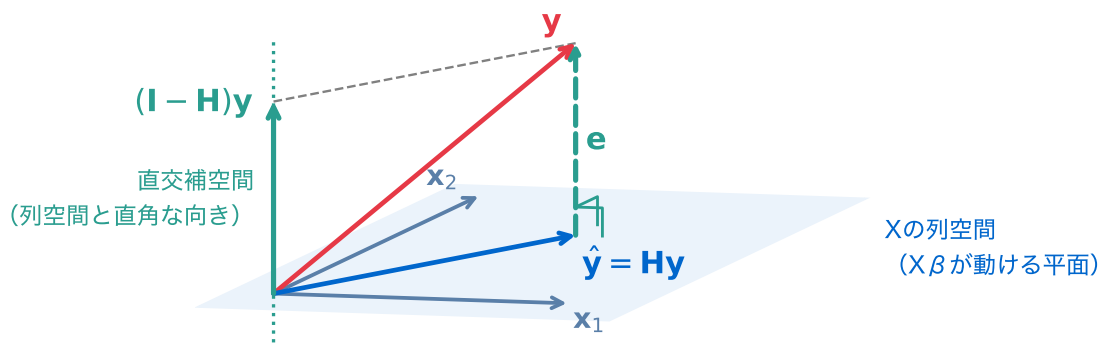
図 11: 観測 \mathbf{y} を、 \mathbf{X} の列空間への影 \hat{\mathbf{y}} = \mathbf{H}\mathbf{y} と、直交補空間(点線)への影 (\mathbf{I} - \mathbf{H})\mathbf{y} = \mathbf{e} に分ける(概念図)。残差 \mathbf{e} は平面に垂直で、どの列とも直交する
