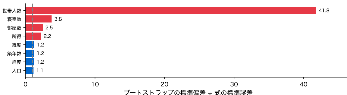
図 24: 地区を復元抽出して 1000 回当てはめ直したときの係数の標準偏差を、式の標準誤差で割った比。破線は 1 (式どおり)
