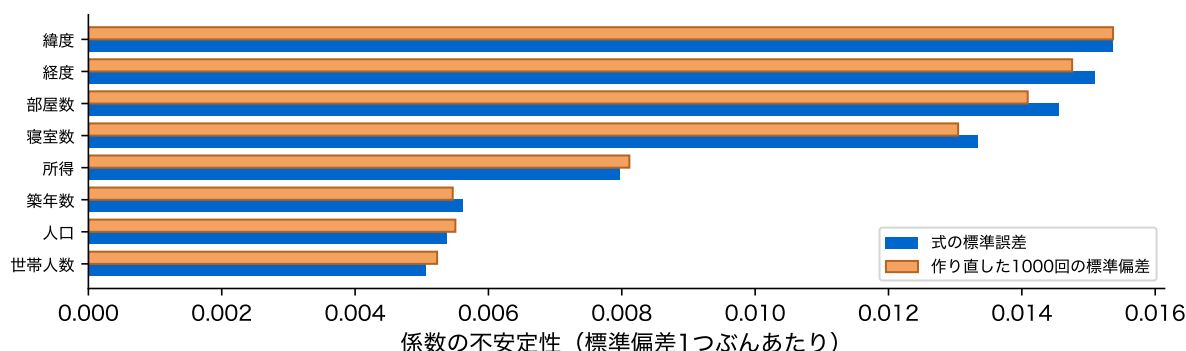
図 20: 係数の不安定性。式 \hat{\sigma}^2(\mathbf{X}^\top \mathbf{X})^{-1} による標準誤差(青)と、 \mathbf{X} を固定して目的変数を 1000 回作り直したときの標準偏差(橙)。標準偏差 1 つぶんあたりに直してある
