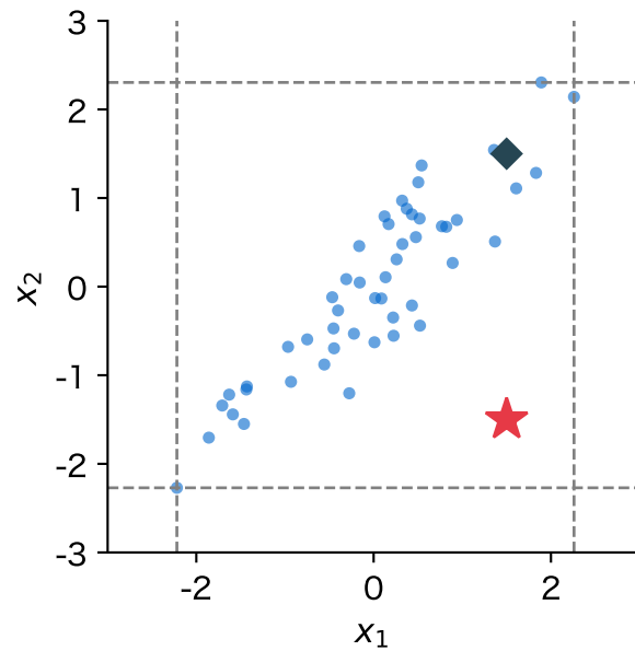
図 16: 相関 0.9 の 2 列(人工データ、50 行)。破線は各列の最小値と最大値。★はどちらの列も範囲の中だが雲の外の点、◆は原点から同じ遠さで雲に沿った点
