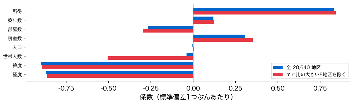
図 26: 全地区で当てはめた係数(青)と、てこ比の大きい 5 地区を除いて当てはめた係数(赤)。標準偏差 1 つぶんあたり
