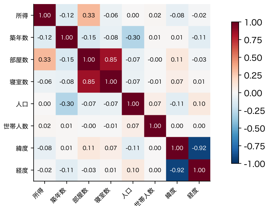
図 19: カリフォルニア住宅データの 8 列の相関行列
