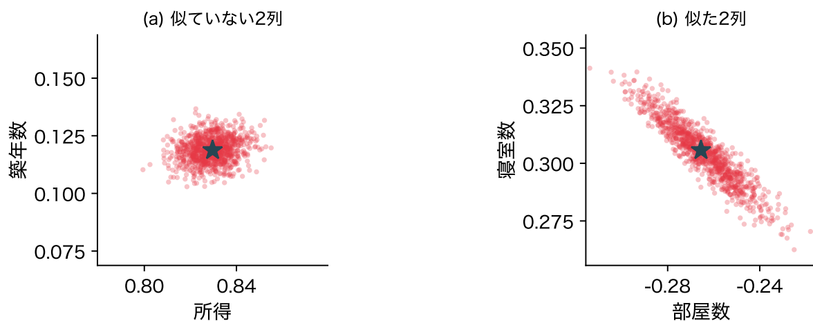
図 21: X を固定して目的変数を 1000 回作り直したときの係数(標準偏差 1 つぶんあたり)。★は全地区で当てはめた値で、2 枚とも★から \pm 0.05 の範囲を描いた。(a) 所得と築年数、(b) 部屋数と寝室数
