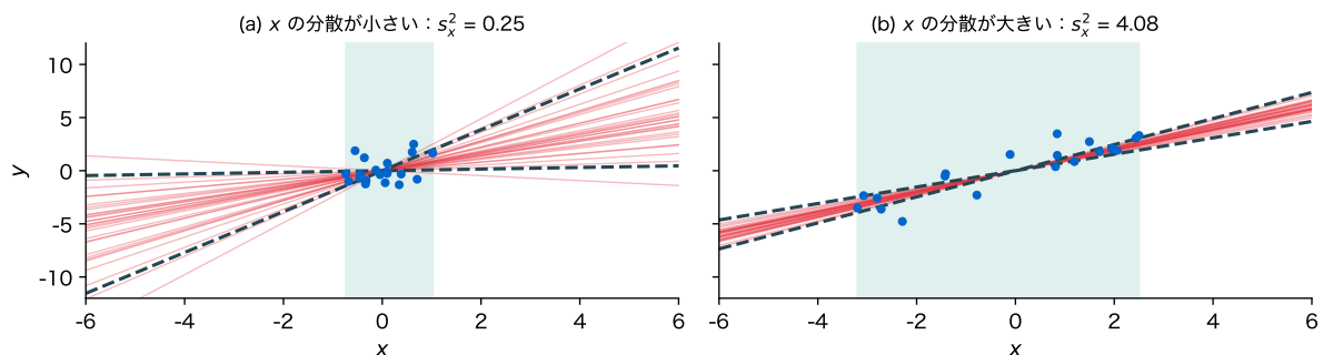
図 6: 人工データで、 x を固定したまま y を 30 回取り直して引いた原点を通る直線(赤)。(a) x の標本分散が小さい、(b) 大きい。青は 1 回ぶんの点、緑はデータのある範囲、破線は予測の \pm 2 標準偏差(後述)
