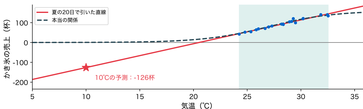
図 15: かき氷の売上と気温(人工データ)。緑は記録のある範囲、赤は記録から引いた直線、破線は本当の関係。 ★は記録にない 10 °C の日の予測
