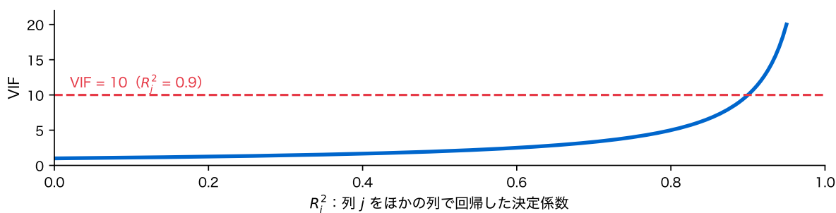
図 9: 分散拡大係数 \text{VIF}_j = 1/(1 - R_j^2) と、目安とされる \text{VIF} = 10 (赤の破線)
