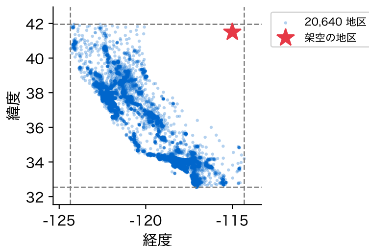
図 27: 地区の緯度と経度と、架空の地区(★)。破線は緯度・経度それぞれの最小値と最大値
