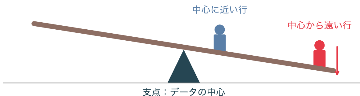
図 13: てこ比のたとえ(概念図)。直線はデータの中心を支点に回る板で、中心から遠い行ほど板を大きく傾ける
