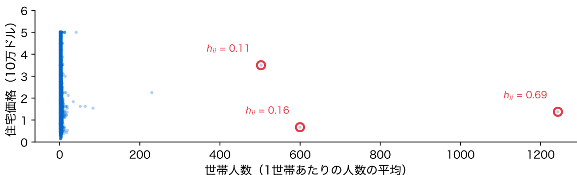
図 25: 世帯人数と住宅価格。赤丸は世帯人数の大きい 3 地区で、数字はそのてこ比
