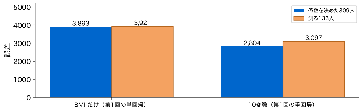
図 9: 第 1 回の 2 つのモデルを、訓練 309 人で係数を決めて、訓練(青)とテスト 133 人(橙)で測った誤差(二乗誤差の平均)
