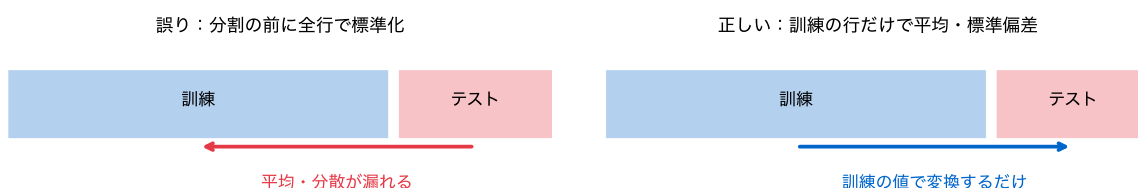
図 8: データリーク。左：分割の前に全行で標準化すると、テストの行の平均・分散が訓練に漏れる。右：訓練の行の値でテストも変換する
