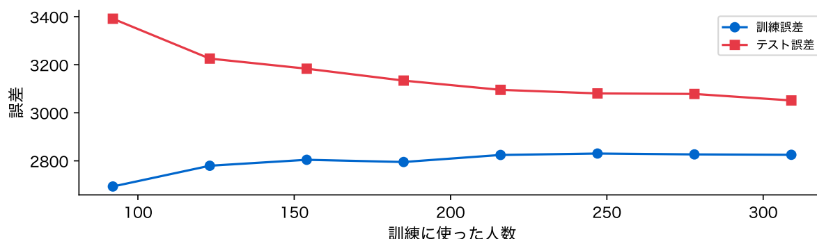
図 11: 学習曲線。訓練に使う人数を増やしたときの訓練誤差(青)とテスト誤差(赤)
