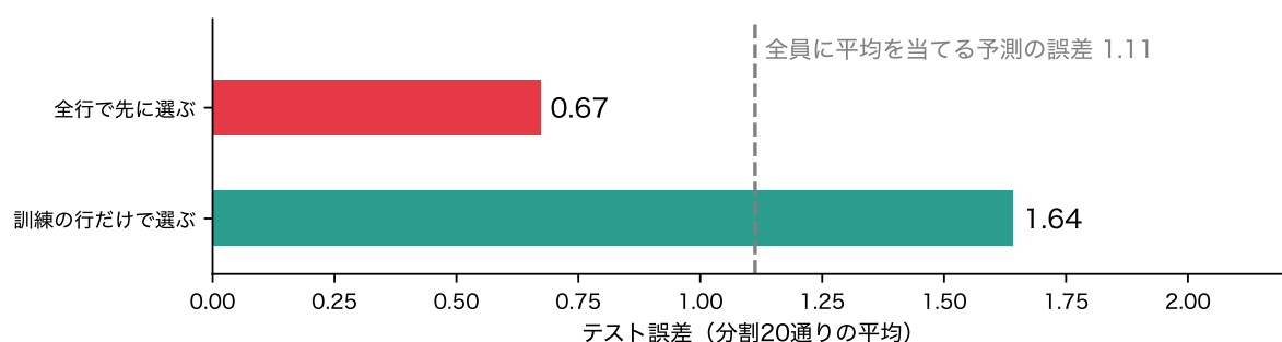
図 12: 目的変数も列もでたらめな人工データで、列を選ぶ行を変えたときのテスト誤差
