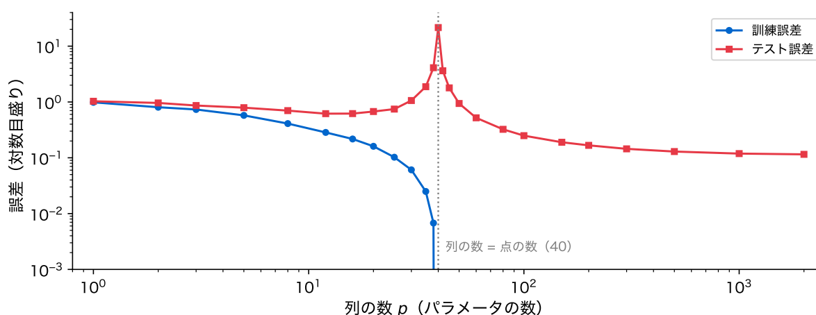
図 13: 人工データでの二重降下。訓練 40 点に、列の数 p を変えて最小二乗法を当てはめたときの訓練誤差(青)とテスト誤差(赤)。 p > 40 では係数のユークリッドノルムが最小の解を使う。 p \geq 40 の訓練誤差は 0 なので描いていない。両軸とも対数目盛り
