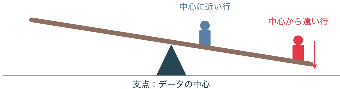
図12: てこ比のたとえ(概念図)。直線はデータの中心を支点に回る板で、中心から遠い行ほど板を大きく傾ける
