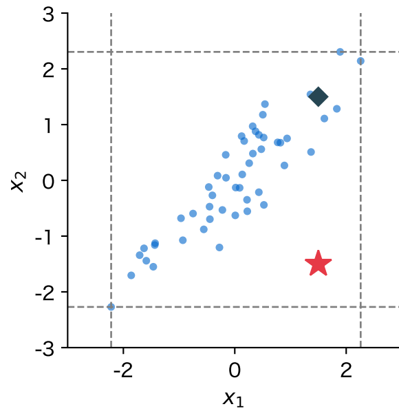
図 15: 相関 0.9 の 2 列(人工データ、50 行)。破線は各列の最小値と最大値。★はどちらの列も範囲の中だが雲の外の点、◆は原点から同じ遠さで雲に沿った点
