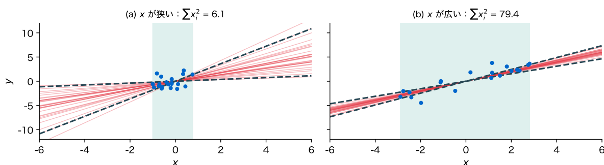
図 5: 人工データで、 x を固定したまま y を 30 回取り直して引いた原点を通る直線(赤)。(a) x が狭い範囲、(b) 広い範囲。青は 1 回ぶんの点、緑はデータのある範囲、破線は予測の \pm 2 標準偏差(後述)
