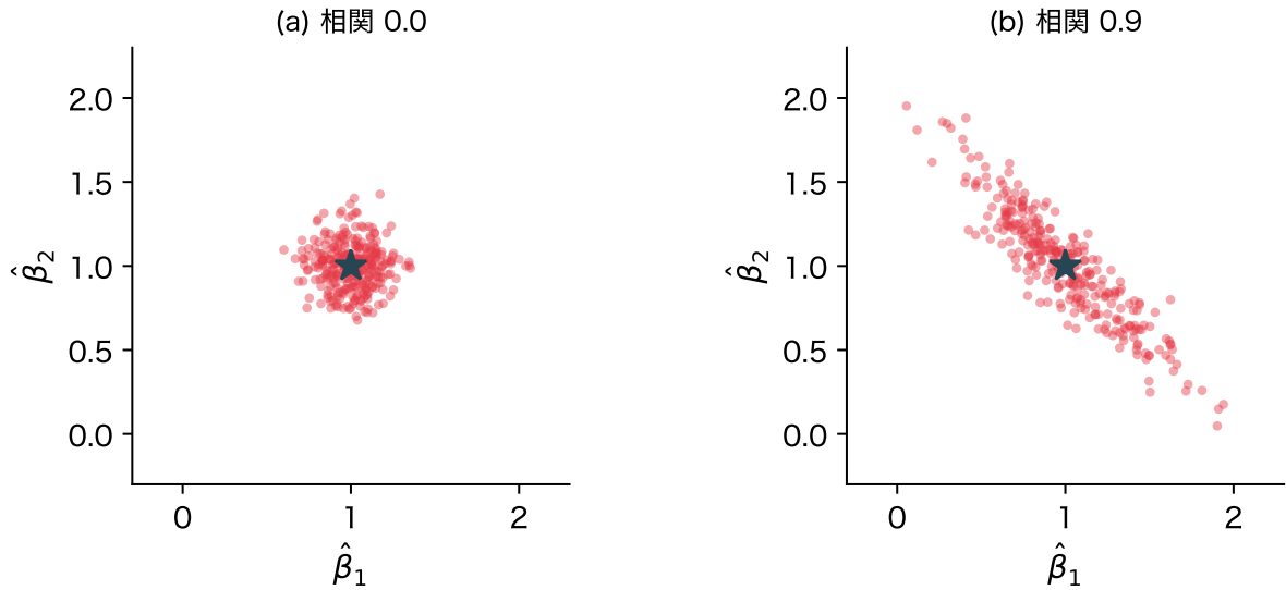
図 7: 人工データで y を 300 回取り直したときの係数の推定値。★は真の値。(a) 2 列の相関が 0、(b) 0.9
