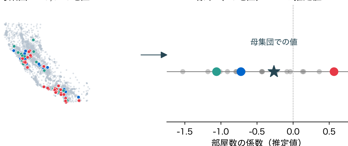
図 3: 母集団と標本と推定値。(左) 20,640 地区を母集団とみたときの 40 地区の標本 3 つ(青・緑・赤)、(右) 標本ごとの部屋数の係数の推定値(灰色は 20 回ぶん)と、母集団での値(★)
