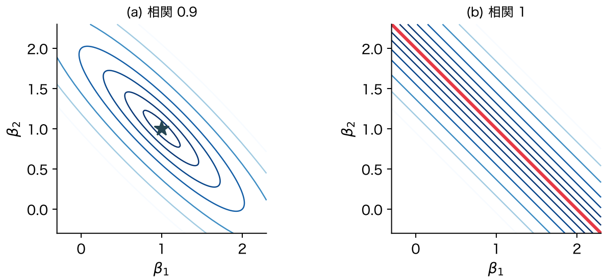
図 16: 2 列の場合の目的関数の等高線(人工データ)。(a) 相関 0.9 では底が 1 点(★)、(b) 相関 1 では底が直線(赤)になり、解が無数にある
