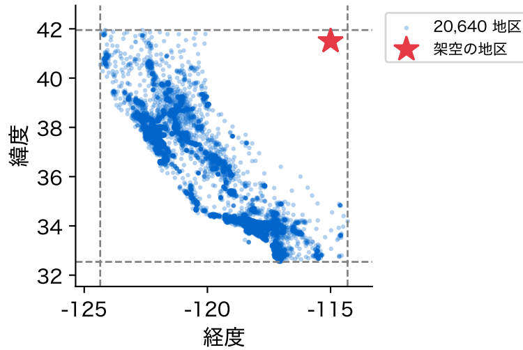
図 25: 地区の緯度と経度と、架空の地区(★)。破線は緯度・経度それぞれの最小値と最大値
