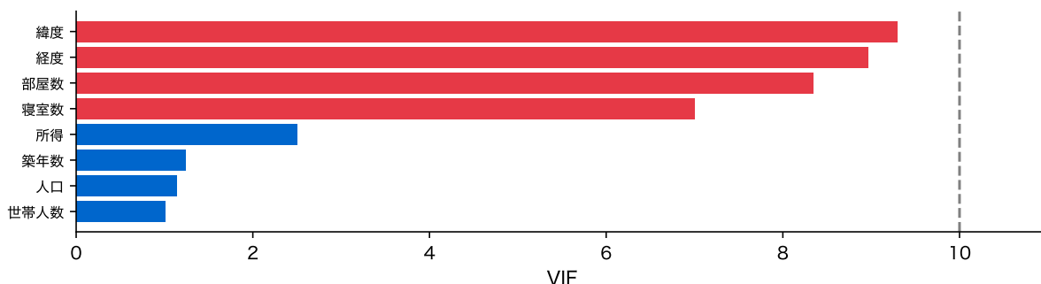
図 21: カリフォルニア住宅データの 8 列の VIF。赤は 5 以上の列、破線は目安とされる VIF = 10
