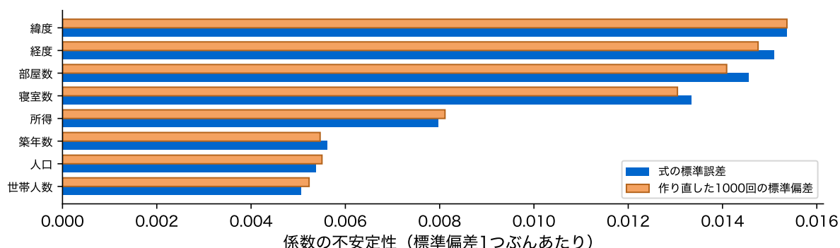
図 19: 係数の不安定性。式 \hat{\sigma}^2(\mathbf{X}^\top \mathbf{X})^{-1} による標準誤差(青)と、 \mathbf{X} を固定して目的変数を 1000 回作り直したときの標準偏差(橙)。標準偏差 1 つぶんあたりに直してある
