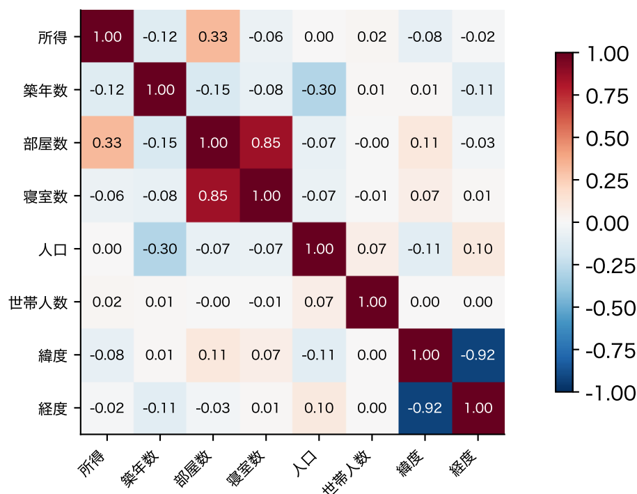
図 18: カリフォルニア住宅データの 8 列の相関行列
