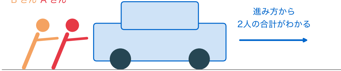
図 6: 共線性のたとえ(概念図)。いつも 2 人で押す車では、進み方から 2 人の力の合計はわかるが、内訳はわからない
