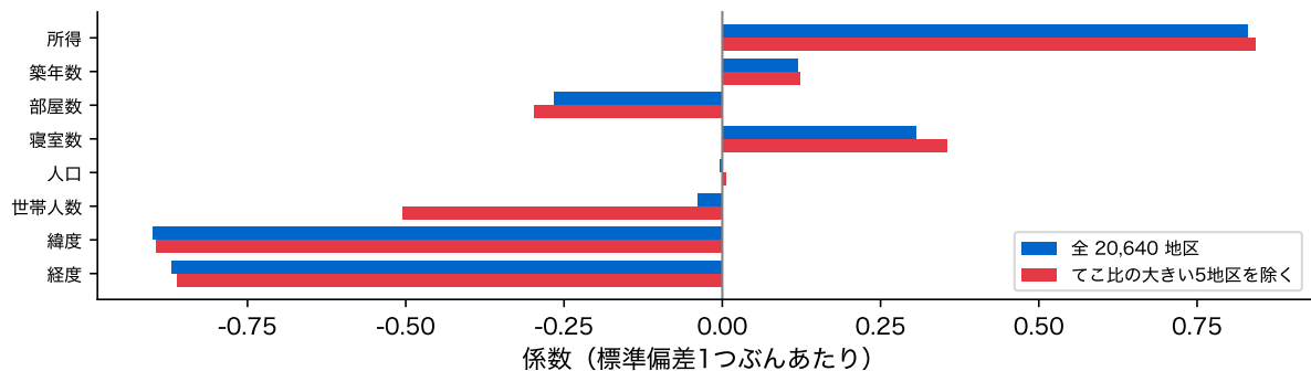
図 24: 全地区で当てはめた係数(青)と、てこ比の大きい 5 地区を除いて当てはめた係数(赤)。標準偏差 1 つぶんあたり
