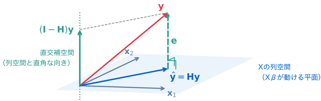
図 10: 観測 \mathbf{y} を、 \mathbf{X} の列空間への影 \hat{\mathbf{y}} = \mathbf{H}\mathbf{y} と、直交補空間(点線)への影 (\mathbf{I} - \mathbf{H})\mathbf{y} = \mathbf{e} に分ける(概念図)。残差 \mathbf{e} は平面に垂直で、どの列とも直交する
