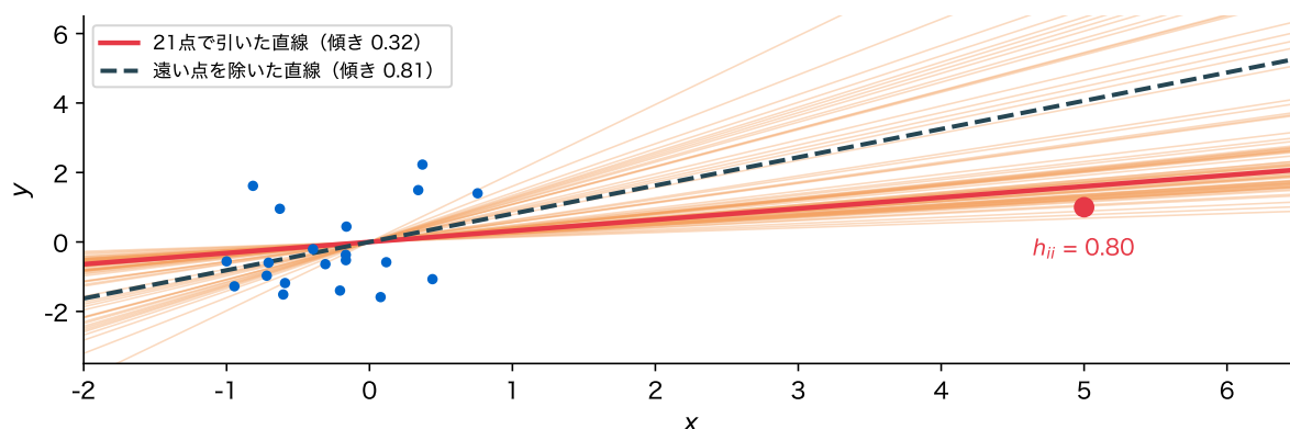
図 13: てこ比の大きい 1 点(人工データ)。青の 20 点に x = 5 の赤の点を足した。赤の実線は 21 点で、黒の破線は赤の点を除いて引いた直線。橙は 21 行を復元抽出して引き直した直線(80 回ぶん)
