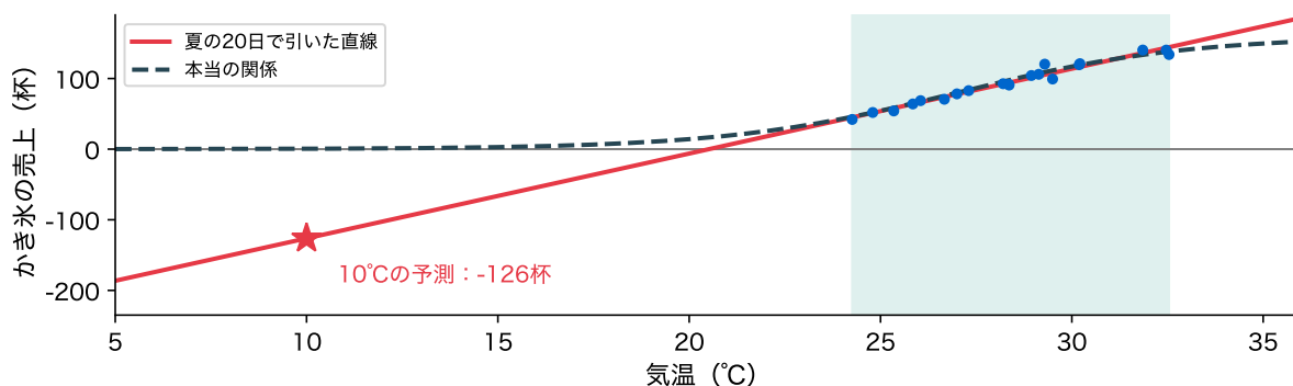
図 14: かき氷の売上と気温(人工データ)。緑は記録のある範囲、赤は記録から引いた直線、破線は本当の関係。 ★は記録にない 10 °C の日の予測
