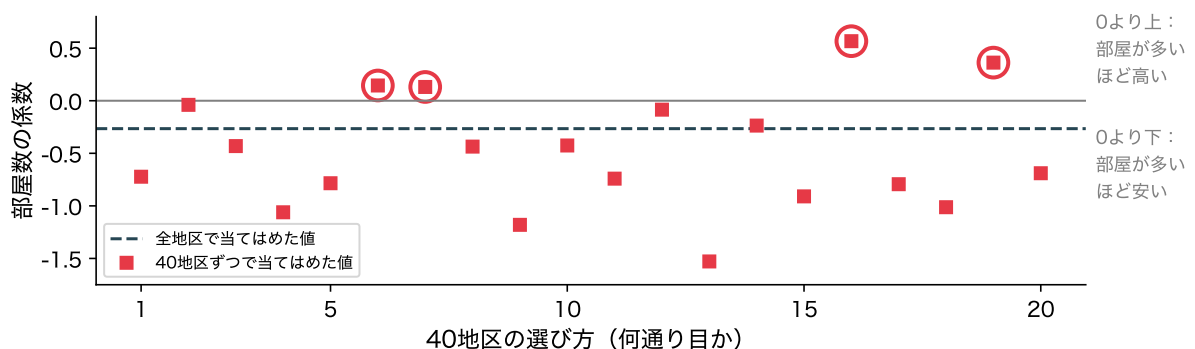
図 2: 20,640 地区から 40 地区を選んで当てはめた部屋数の係数(標準偏差 1 つぶんあたり、20 回)。破線は全地区で当てはめた値、○は符号が逆になった回
