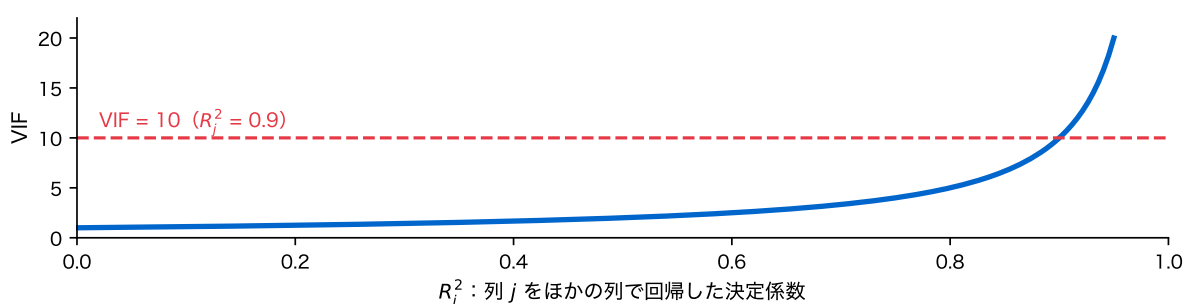
図 8: 分散拡大係数 VIF_j = 1/(1 - R_j^2) と、目安とされる VIF = 10 (赤の破線)
