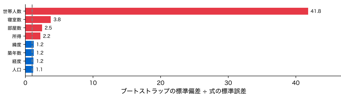
図 22: 地区を復元抽出して 1000 回当てはめ直したときの係数の標準偏差を、式の標準誤差で割った比。破線は 1 (式どおり)
