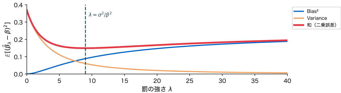
図 6: 1 変数のリッジ回帰の係数の二乗誤差 (9) 式と、その \text{Bias}^2 (青)・ \text{Variance} (橙)。破線は底の位置 \lambda = \sigma^2/\beta^2 (人工データの設定で計算)
