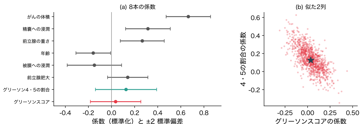
図 1: 前立腺がんのデータで、97 人のブートストラップ 1000 回から求めた係数のばらつき (標準化した単位)。(a) 全員で当てはめた係数と \pm 2 標準偏差。赤がグリーソンスコア、緑がグリーソン 4・5 の割合。(b) その 2 つの係数の 1000 回ぶん。★は全員で当てはめた値
