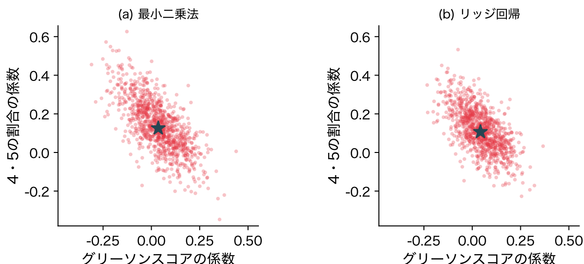
図 17: ブートストラップ 1000 回でのグリーソンスコアとグリーソン 4・5 の割合の係数(標準化した単位)。(a) 最小二乗法、(b) CV で選んだ \lambda のリッジ回帰。★は全員で当てはめた値
