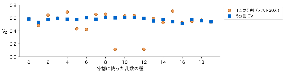
図 18: 分割の乱数を 20 通り変えたときの R^2 。1 回の分割(訓練 67 人・テスト 30 人、橙)と、5 分割 CV (青)
