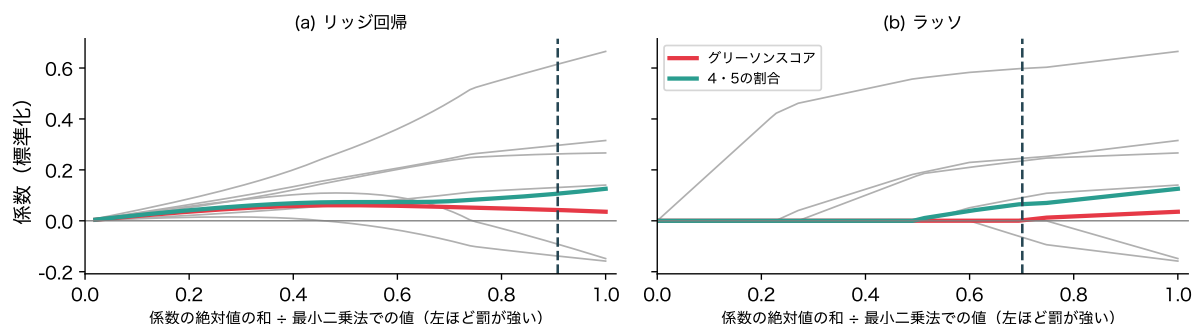
図 15: 前立腺がんのデータの係数の道筋(標準化した単位)。(a) リッジ回帰、(b) ラッソ。赤がグリーンソスコア、緑がグリーンソン 4・5 の割合、灰はほかの 6 変数。破線は 5 分割 CV で選んだ罰の強さ
