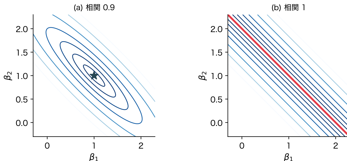
図 15: 2 列の場合の目的関数の等高線(人工データ)。(a) 相関 0.9 では底が 1 点(★)、(b) 相関 1 では底が直線(赤)になり、解が無数にある
