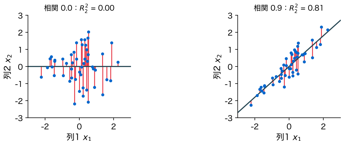
図 11: 列 2 を列 1 と切片で回帰したときの残差 \tilde{x}_2 (赤)。(a) 相関 0 の 2 列、(b) 相関 0.9 の 2 列(人工データ、50 行)。似た列では、ほかの列で説明できない部分がわずかしかなかった
