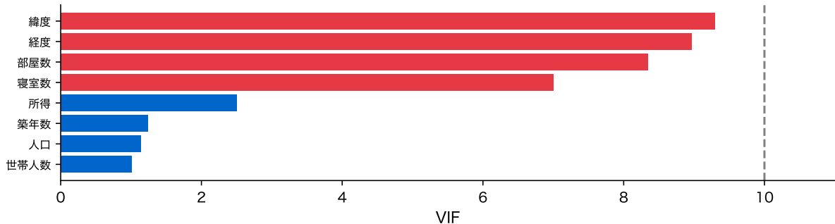
図 20: カリフォルニア住宅データの 8 列の VIF。赤は 5 以上の列、破線は目安とされる VIF = 10
