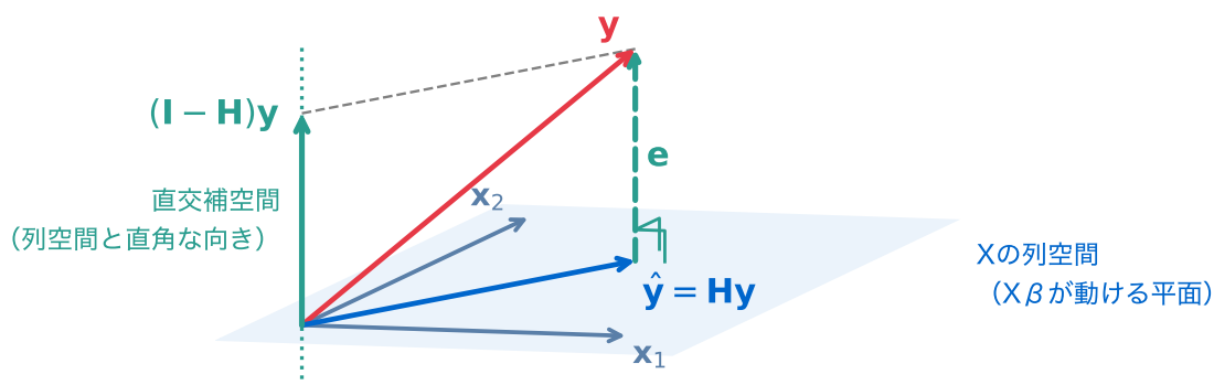
図 7: 観測 y を、 X の列空間への影 \hat{y} = Hy と、直交補空間(点線)への影 (I-H)y = e に分ける(概念図)。残差 e は平面に垂直で、どの列とも直交する
