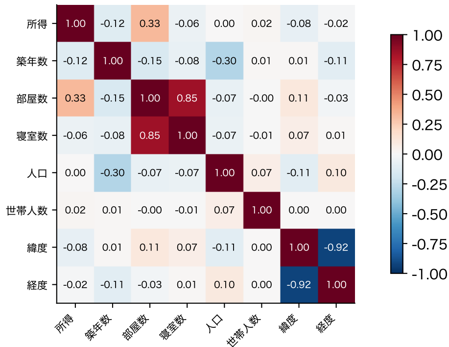
図 17: カリフォルニア住宅データの 8 列の相関行列
