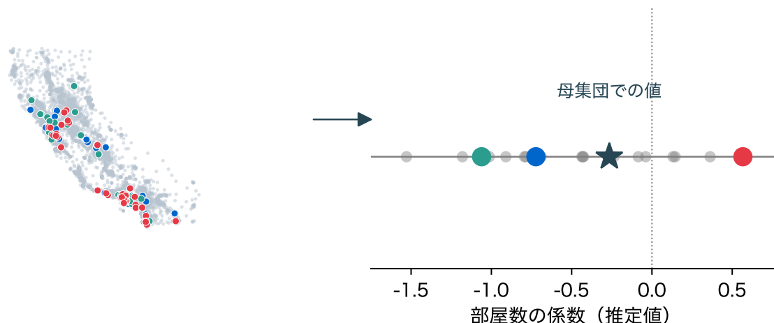
図 21: 20,640 地区を母集団とみなしたときの、40 地区の標本 3 つ(左、青・緑・赤)と、標本ごとの部屋数の係数の推定値(右、灰色は 20 回ぶん)。★は全地区での値、0 より右は符号が逆
