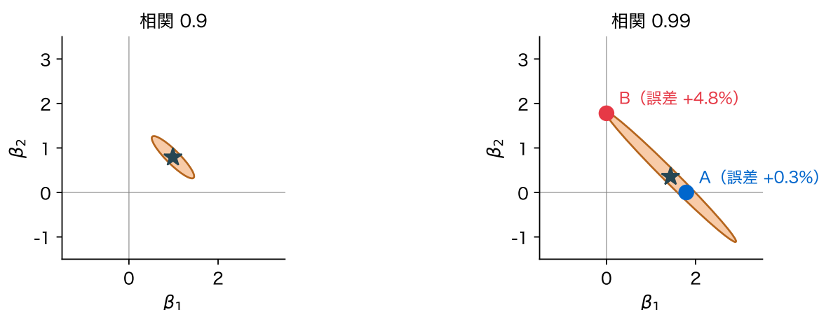
図 22: 羅生門集合(人工データ、50 行)。訓練の二乗誤差が最小(★)から 5% 以内の係数の組(橙)。(左) 相関 0.9、(右) 相関 0.99。A は列 1 だけ、B は列 2 だけを使うモデル
