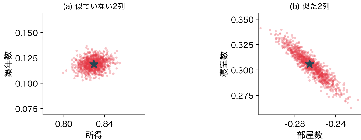
図 19: \mathbf{X} を固定して目的変数を 1000 回作り直したときの係数(標準偏差 1 つぶんあたり)。★は全地区で当てはめた値で、2 枚とも★から \pm 0.05 の範囲を描いた。(a) 所得と築年数、(b) 部屋数と寝室数
