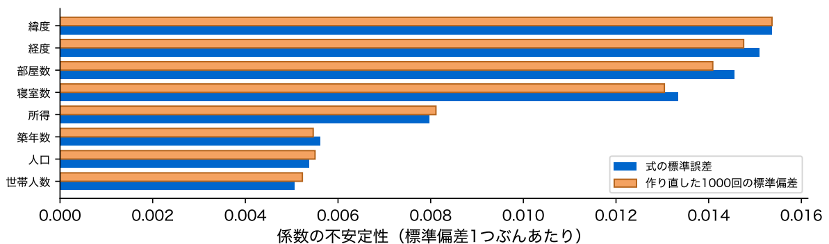
図 18: 係数の不安定性。式 \hat{\sigma}^2(\mathbf{X}^\top \mathbf{X})^{-1} による標準誤差(青)と、 \mathbf{X} を固定して目的変数を 1000 回作り直したときの標準偏差(橙)。標準偏差 1 つぶんあたりに直してある
