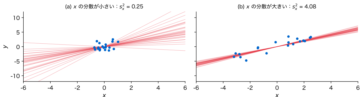
図 8: 人工データで、 x を固定したまま y を 30 回取り直して引いた原点を通る直線(赤)。(a) x の標本分散が小さい、(b) 大きい。青は 1 回ぶんの点
