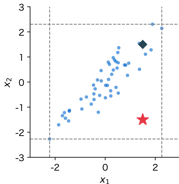
図 9: 相関 0.9 の 2 列(人工データ、50 行)。破線は各列の最小値と最大値。★はどちらの列も範囲の中だが雲の外の点、◆は原点から同じ遠さで雲に沿った点
