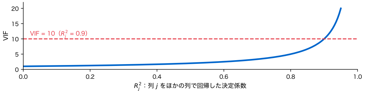
図 5: 分散拡大係数 VIF_j = 1/(1 - R_j^2) と、目安とされる VIF = 10 (赤の破線)
