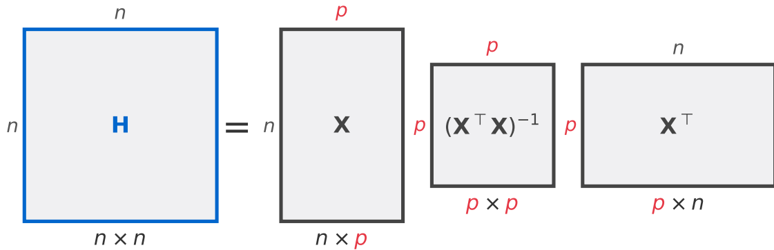
図 6: 射影行列 \mathbf{H} = \mathbf{X}(\mathbf{X}^\top \mathbf{X})^{-1} \mathbf{X}^\top の大きさ(概念図)。箱の縦は行数、横は列の数。赤は掛け算でそろった次元
