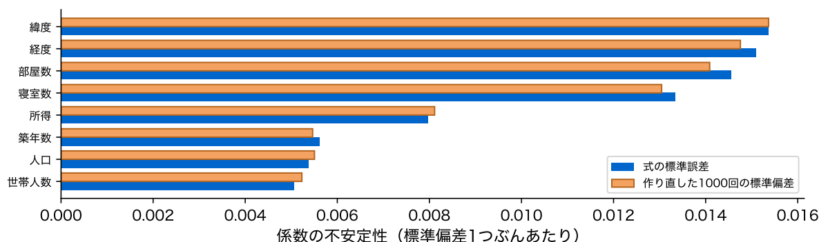
図 12: 係数の不安定性。式 \hat{\sigma}^2(\mathbf{X}^T \mathbf{X})^{-1} による標準誤差(青)と、 \mathbf{X} を固定して目的変数を 1000 回作り直したときの標準偏差(橙)。標準偏差 1 つぶんあたりに直してある
