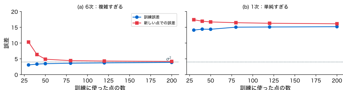
図 7: 人工データの学習曲線。(a) 6次(複雑すぎる)、(b) 1次(単純すぎる)。点線は \sigma^2
