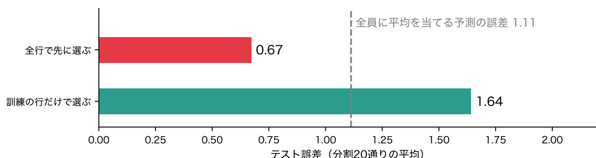
図 13: 目的変数も列もでたらめな人工データで、列を選ぶ行を変えたときのテスト誤差
