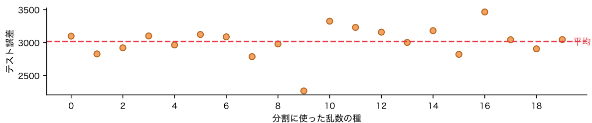
図 15: 第 1 回の 10 変数のモデルを、分割の乱数だけ変えて測り直したテスト誤差(20 通り)
