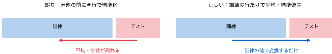
図 9: データリーク。左：分割の前に全行で標準化すると、テストの行の平均・分散が訓練に漏れる。右：訓練の行の値でテストも変換する
