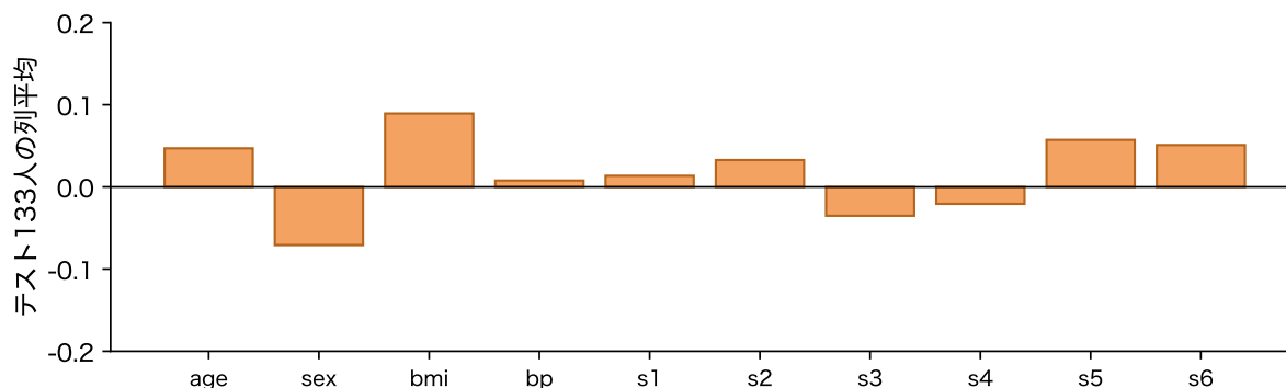
図 11: 訓練 309 人の平均・標準偏差で標準化したテスト 133 人の、列ごとの平均
