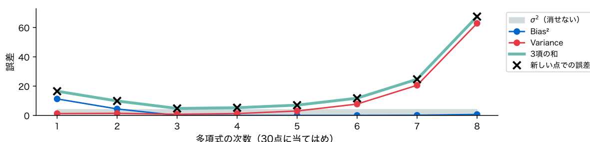
図 6: 人工データでのバイアス・バリアンス分解。30 点の訓練データを 300 回取り直して計算した 3 項と、その和(緑)、新しい点で直接測った誤差(x)
