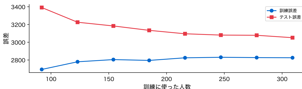
図 12: 学習曲線。訓練に使う人数を増やしたときの訓練誤差(青)とテスト誤差(赤)
