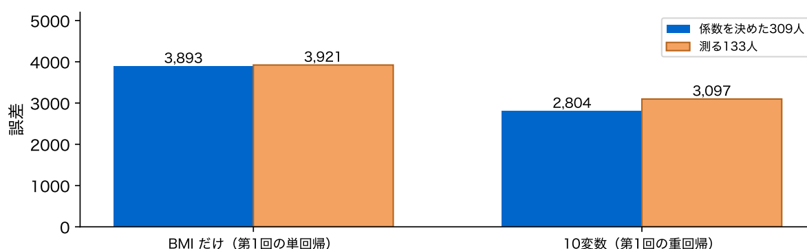
図 10: 第 1 回の 2 つのモデルを、訓練 309 人で係数を決めて、訓練(青)とテスト 133 人(橙)で測った誤差(二乗誤差の平均)
