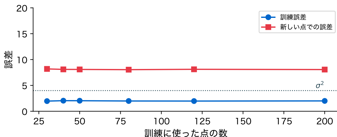
図 8: 人工データで、無関係な列を足して係数の数を点の数の半分にしたときの訓練誤差と新しい点での誤差。点線は \sigma^2
