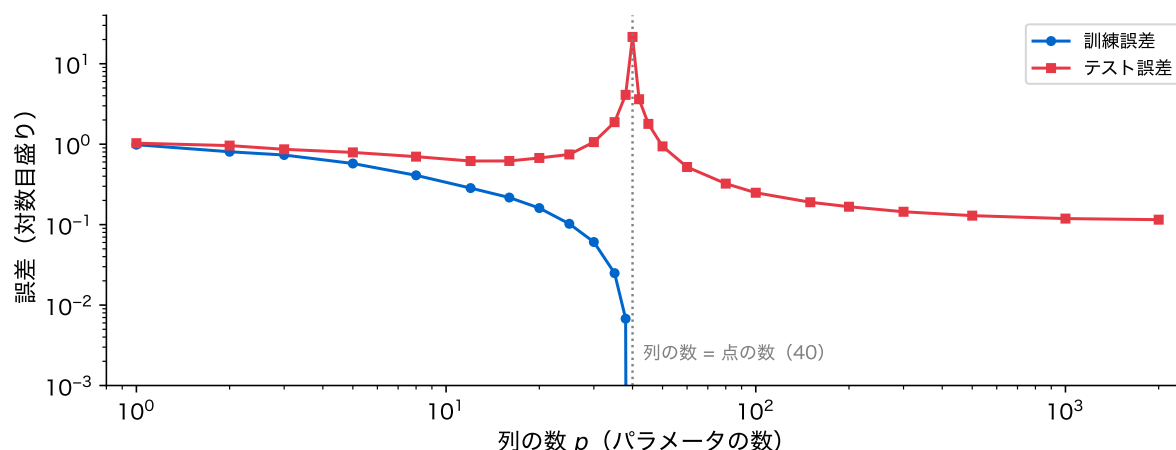
図 14: 人工データでの二重降下。訓練 40 点に、列の数 p を変えて最小二乗法を当てはめたときの訓練誤差(青)とテスト誤差(赤)。 p > 40 では係数のユークリッドノルムが最小の解を使う。 p \geq 40 の訓練誤差は 0 なので描いていない。両軸とも対数目盛り
