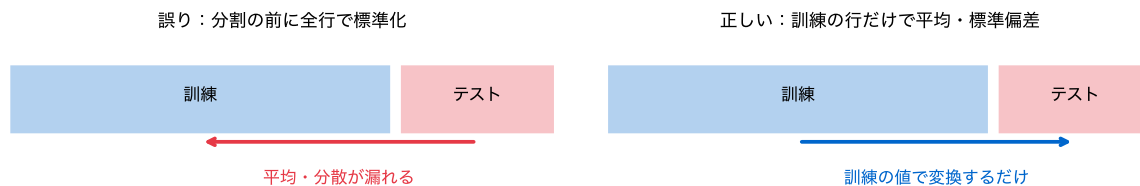
図 11: データリーク。左：分割の前に全行で標準化すると、テストの行の平均・分散が訓練に漏れる。右：訓練の行の値でテストも変換する
