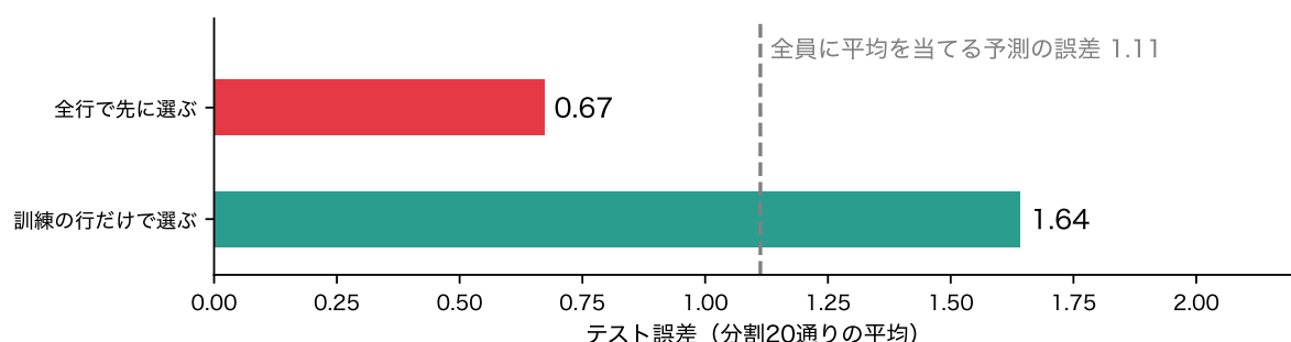
図 15: 目的変数も列もでたらめな人工データで、列を選ぶ行を変えたときのテスト誤差
