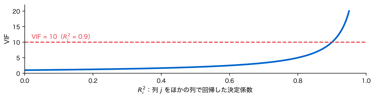
図 9: 分散拡大係数 VIF_j = 1/(1 - R_j^2) と、目安とされる VIF = 10 (赤の破線)
