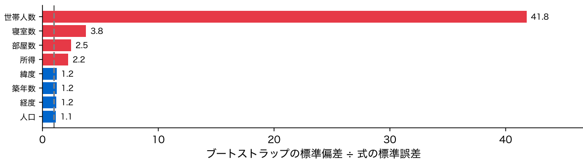
図 23: 地区を復元抽出して 1000 回当てはめ直したときの係数の標準偏差を、式の標準誤差で割った比。破線は 1 (式どおり)
