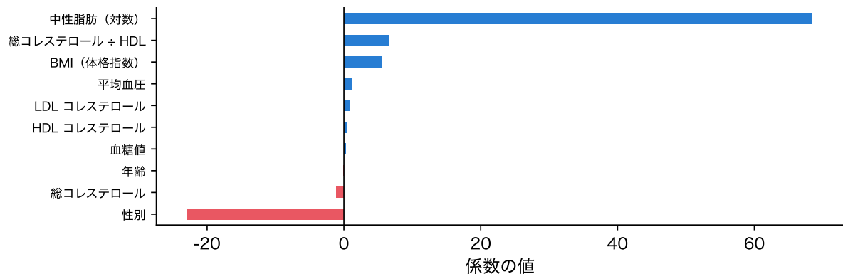
図 13: 重回帰の係数(元の単位のまま)
