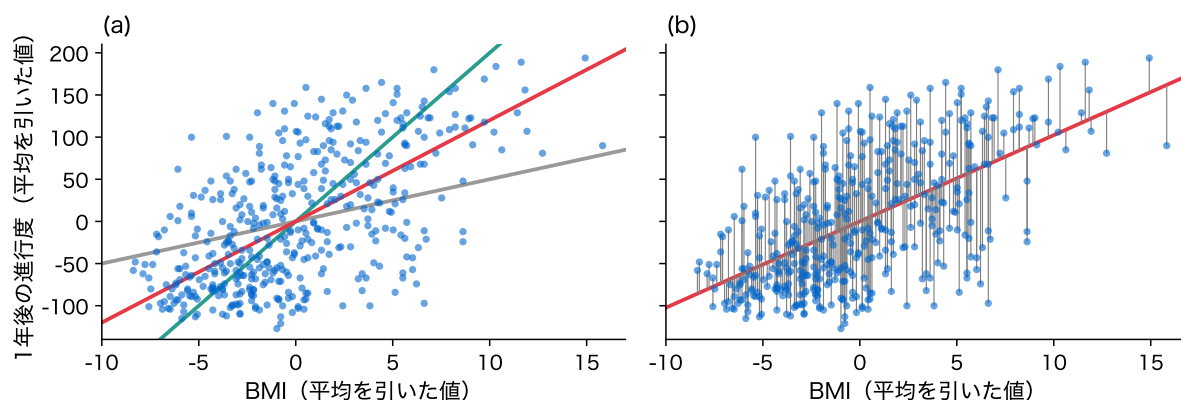
図 3: BMI と 1 年後の進行度(患者 442 人、どちらも平均を引いた値)。(a) 傾きの違う直線、(b) 最小二乗法で選んだ直線と各点の縦のずれ
