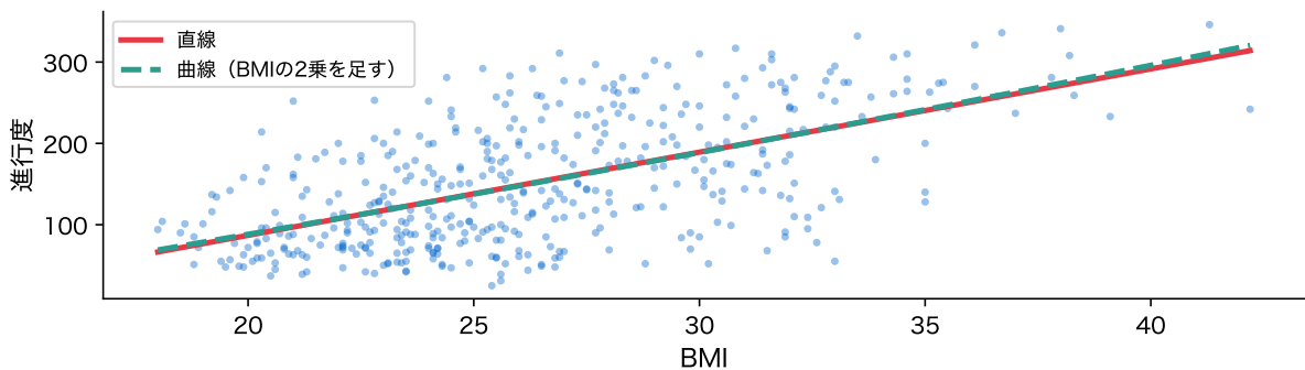
図 12: BMI と進行度。最小二乗法で当てはめた直線(赤)と、BMI の 2 乗の列を足した曲線(緑の破線)
