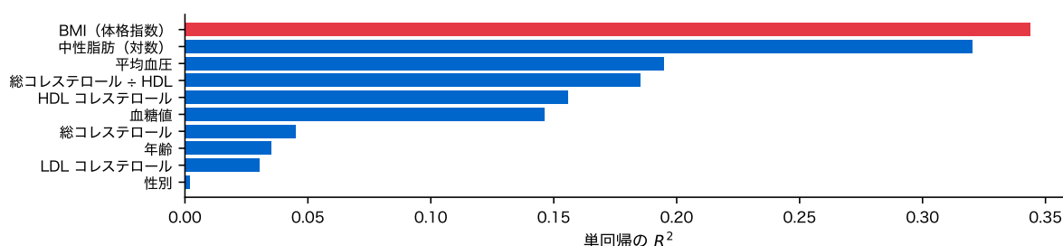
図 10: 説明変数を 1 つずつ使った単回帰の決定係数
