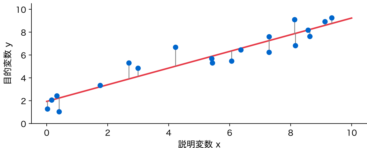
図 1: 最小二乗法の説明によく使われる図
