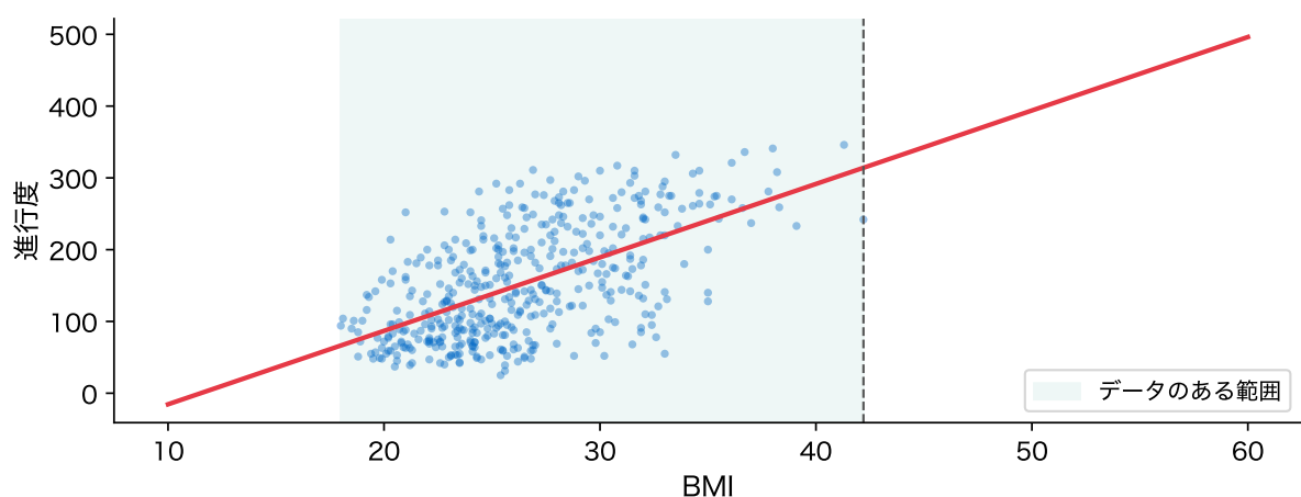
図 14: BMI だけの単回帰の直線を、データのある範囲(緑)の外まで延ばしたもの
