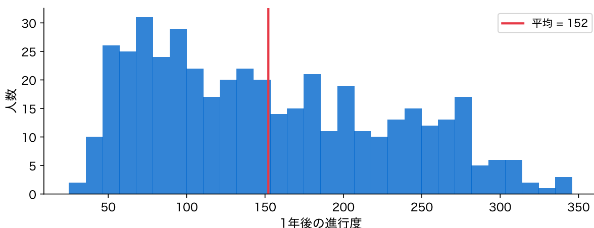
図 9: 目的変数(1 年後の進行度)の分布。赤線は平均
