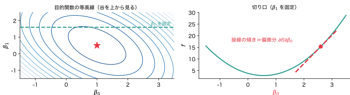
図 6: 係数が 2 つのときの目的関数(概念図)。左:等高線と、 \beta_1 を固定した切り口(緑の破線)。右:その切り口の放物線と、接線の傾き(偏微分)
