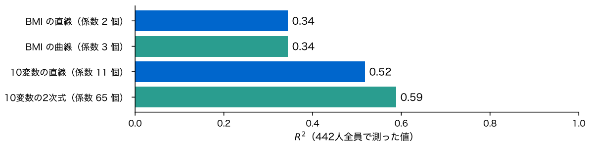
図 11: 同じ最小二乗法で、モデル(データ行列の列)だけを替えた 4 つのモデルの決定係数。442 人全員で当てはめて測った値
