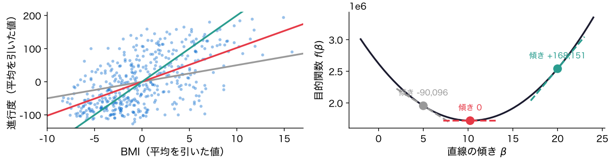
図 5: 左: 傾きの違う 3 本の直線。右: 傾き \beta を動かしたときの目的関数 f(\beta) と、3 本の直線に対応する点での接線
