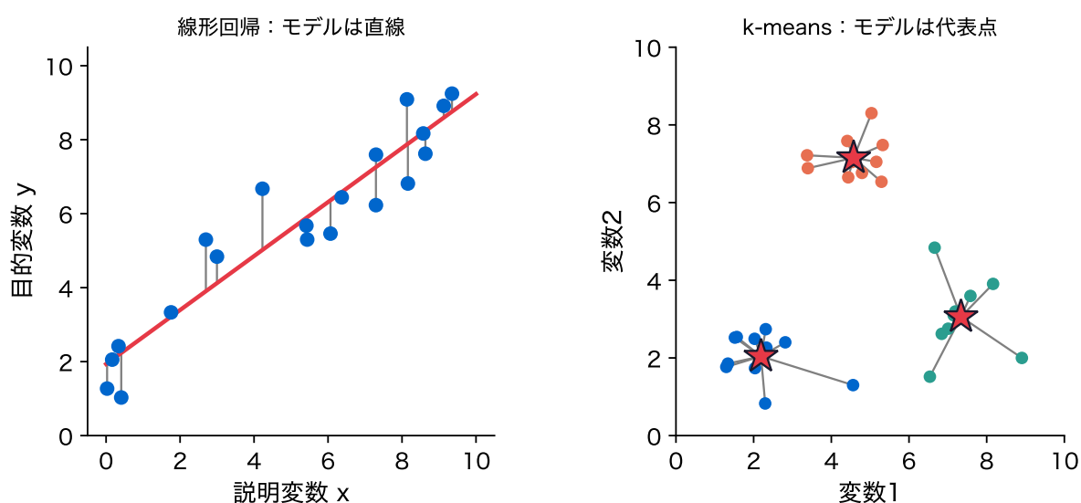
図 8: 同じ推定法、違うモデル。左：線形回帰(誤差は直線への縦の線)。右：k-means (誤差は群の代表点★への線)。どちらも誤差の二乗和を最小にする
