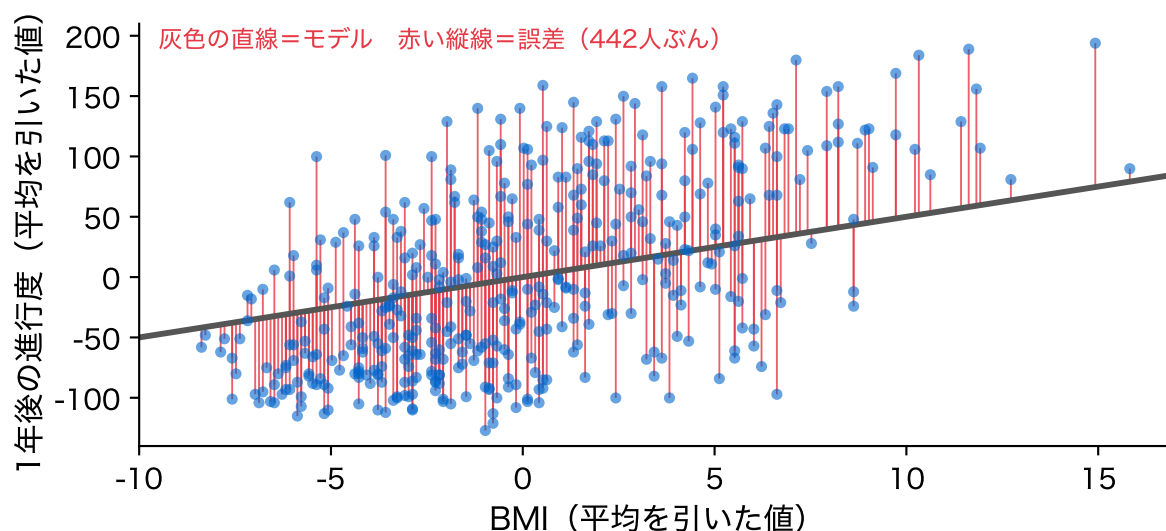
図 4: データ=モデル+誤差。傾き 5 の直線 (灰色) をモデルとしたときの、442 人ぶんの誤差 (赤い縦線)
