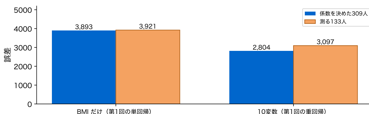
図 8: 第 1 回の 2 つのモデルを、訓練 309 人で係数を決めて、訓練(青)とテスト 133 人(橙)で測った誤差(二乗誤差の平均)
