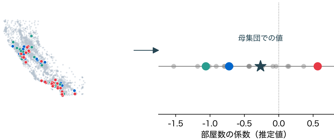
図 20: 20,640 地区を母集団とみなしたときの、40 地区の標本 3 つ(左、青・緑・赤)と、標本ごとの部屋数の係数の推定値(右、灰色は 20 回ぶん)。★は全地区での値、0 より右は符号が逆
