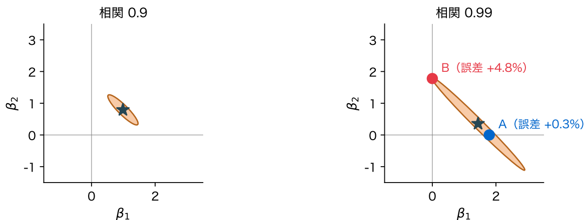
図 21: 羅生門集合(人工データ、50 行)。訓練の二乗誤差が最小(★)から 5% 以内の係数の組(橙)。(左) 相関 0.9、(右) 相関 0.99。A は列 1 だけ、B は列 2 だけを使うモデル
