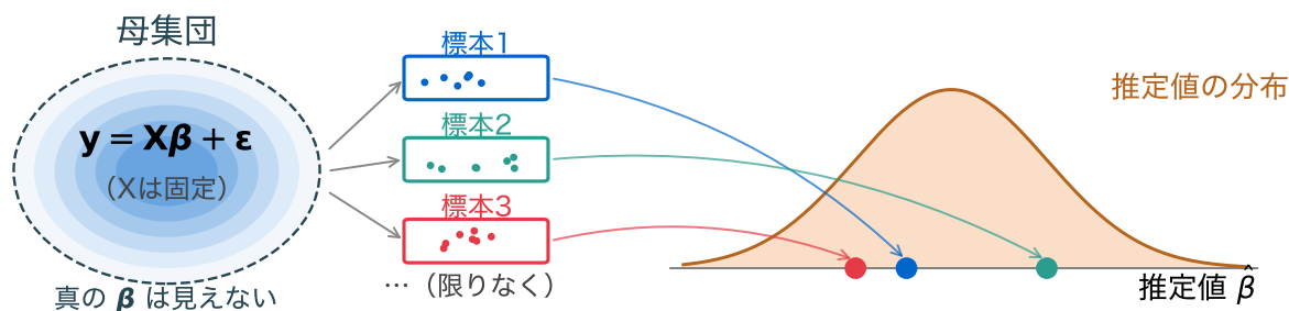
図3: 母集団と標本と推定値(概念図)。母集団 y = X\beta + \epsilon ( X は固定) から標本を取り出すたびに推定値が1つ決まり、限りなく取り直すと推定値の分布になる。真の \beta は見えない
