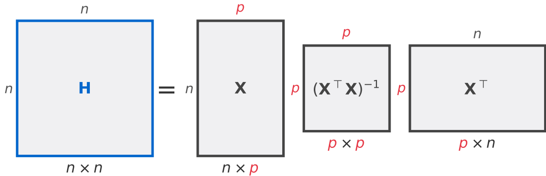
図 8: 射影行列 \mathbf{H} = \mathbf{X}(\mathbf{X}^\top \mathbf{X})^{-1} \mathbf{X}^\top の大きさ(概念図)。箱の縦は行の数、横は列の数。赤は掛け算でそろう次元
