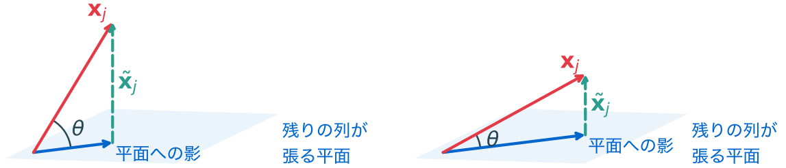
図 12: 共線性の幾何(概念図)。平均を引いた列 \mathbf{x}_j (赤)を、残りの列が張る平面への影(青)と、直交補空間への影 \tilde{\mathbf{x}}_j (緑)に分ける。平面とのなす角 \theta が小さいほど \tilde{\mathbf{x}}_j は短く、 VIF_j = 1/\sin^2\theta は大きい
