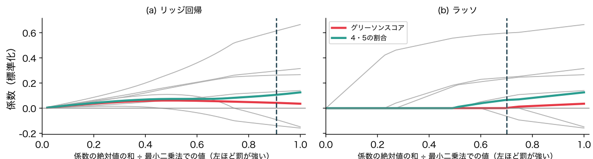
図 16: 前立腺がんのデータの係数の道筋(標準化した単位)。(a) リッジ回帰、(b) ラッソ。赤がグリーンスコア、緑がグリーンソン 4・5 の割合、灰はほかの 6 変数。破線は 5 分割 CV で選んだ罰の強さ
