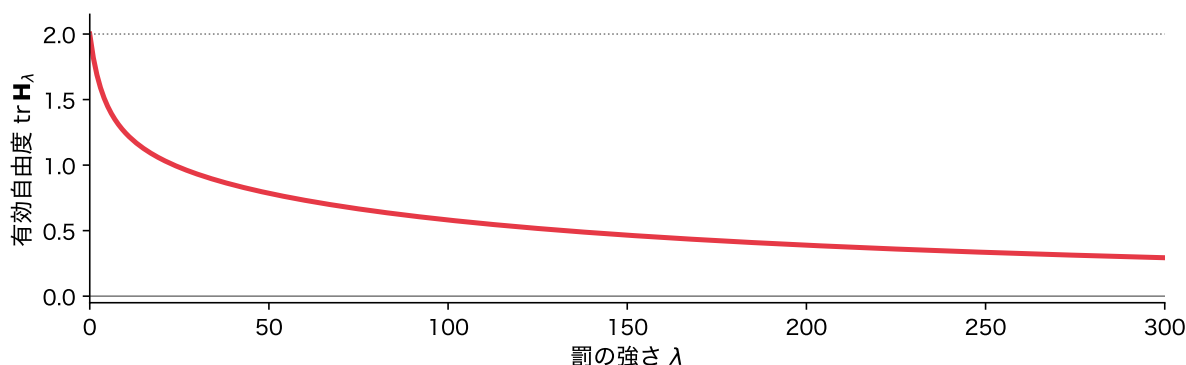
図 12: 麺の量とスープの量の 2 列(人工データ)での、罰の強さ \lambda に対するリッジ回帰の有効自由度
