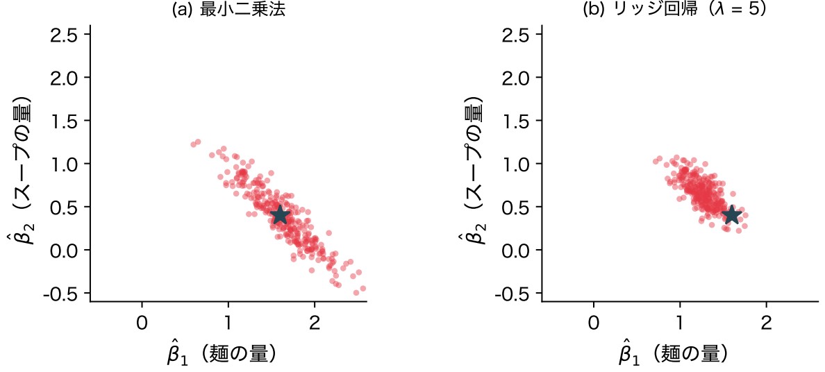
図 7: 麺の量とスープの量(相関 0.92)の 2 列で y を 300 回取り直したときの係数(人工データ)。(a) 最小二乗法、(b) リッジ回帰。★は真の値
