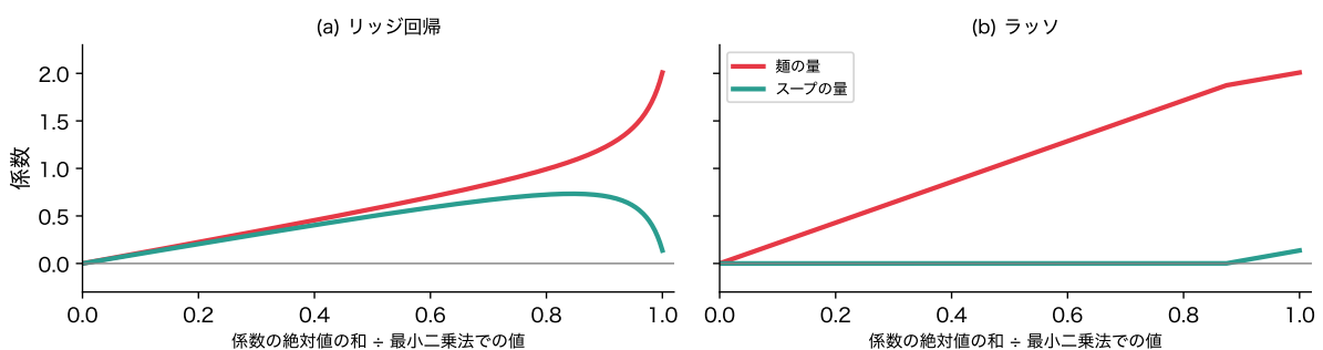
図 11: 麺の量とスープの量(相関 0.92)の 2 列での係数の道筋(人工データ)。(a) リッジ回帰、(b) ラッソ。横軸は係数の絶対値の和を最小二乗法での値で割った比で、右端が最小二乗法
