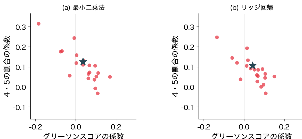
図 18: 訓練・テストへの分け方 20 通りでのグリーンスコアとグリーンソン 4・5 の割合の係数(標準化した単位)。(a) 最小二乗法、(b) CV で選んだ \lambda のリッジ回帰。★は全員で当てはめた値
