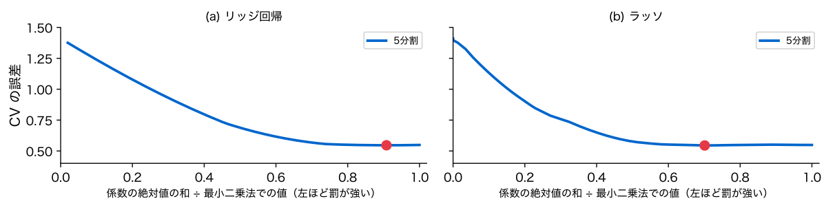
図 17: 罰の強さに対する CV の誤差(二乗平均)。(a) リッジ回帰、(b) ラッソ(どちらも 5 分割)。赤は選んだ強さ
