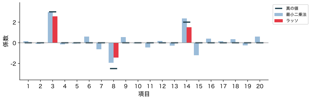
図 10: 40 杯・20 項目の人工データで、効くのは 3 項目だけ(黒の横線が真の値)。最小二乗法(水色)の係数は効かない 17 項目でも 0 にならないが、ラッソ(赤)は効く 3 項目だけを残す
