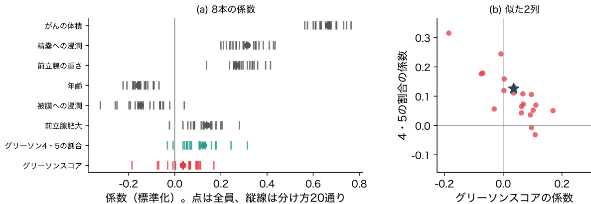
図 1: 前立腺がんのデータで、訓練・テストへの分け方を 20 通り変えて当てはめた係数(標準化した単位)。(a) 全員で当てはめた係数(点)と 20 通りの係数(縦線)。赤がグリーソンスコア、緑がグリーソン 4・5 の割合。(b) その 2 つの係数の 20 通りぶん。★は全員で当てはめた値
