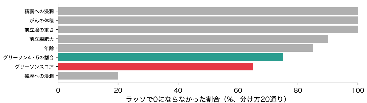
図 20: 訓練・テストへの分け方 20 通りで、CV で選んだ強さのラッソが係数を 0 にしなかった割合。赤がグリーソンスコア、緑がグリーソン 4・5 の割合
