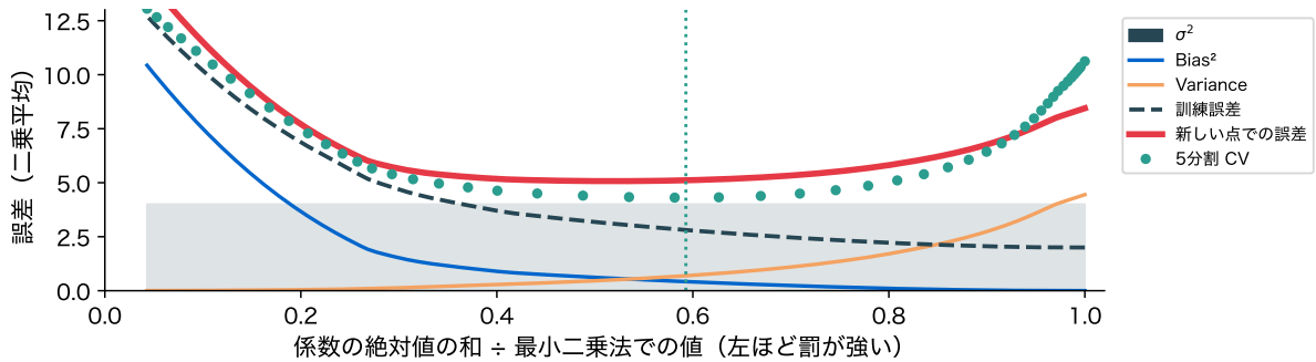
図 15: 人工データ (40 行・20 列) でのリッジ回帰の誤差を、係数の絶対値の和の比 (右端が最小二乗法) に対して描いたもの。訓練誤差 (破線)、新しい点での誤差 (赤) とその \text{Bias}^2 \cdot \text{Variance} \cdot \sigma^2 、1 回ぶんのデータで計算した 5 分割 CV (緑の点。点線は選んだ所)
