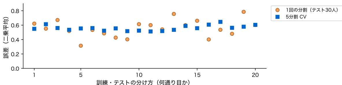
図 19: 訓練・テストへの分け方を 20 通り変えたときの誤差(二乗平均)。1 回の分割(訓練 67 人・テスト 30 人、橙)と、5 分割 CV (青)
