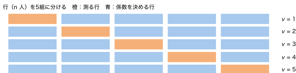
図 14: 5 分割 CV の分け方(概念図)。各回(行)で橙の組を測り、青の組で係数を決める
