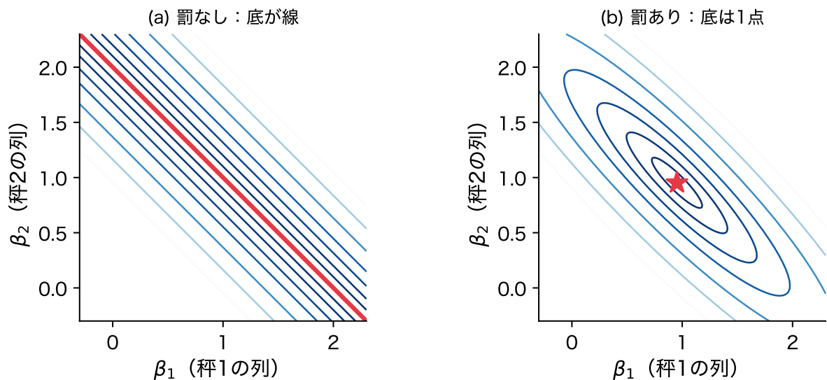
図 4: 同じ麵の量を 2 台の秤で量った相関 1 の 2 列の目的関数の等高線(人工データ)。(a) 罰なしでは底が直線(赤)、(b) 罰を足すと底は 1 点(赤の★)に決まる
