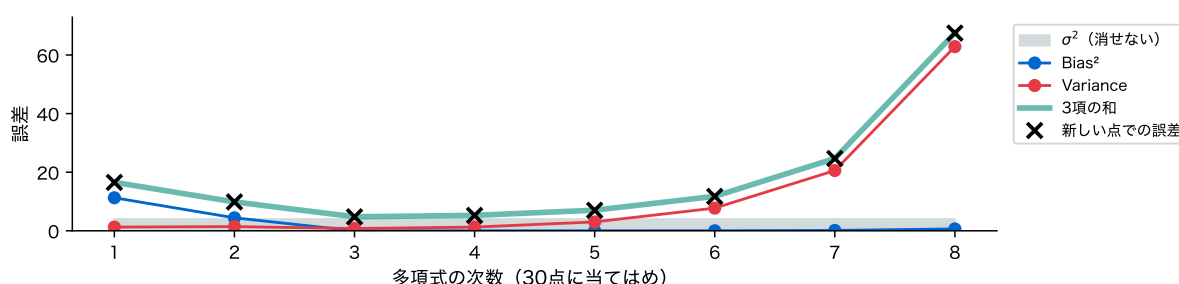
図 6: 人工データでのバイアス・バリエンス分解。30 点の訓練データを 300 回取り直して計算した 3 項と、その和(緑)、新しい点で直接測った誤差(x)
