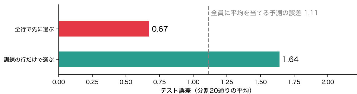
図 12: 目的変数も列もでたらめな人工データで、列を選ぶ行を変えたときのテスト誤差
