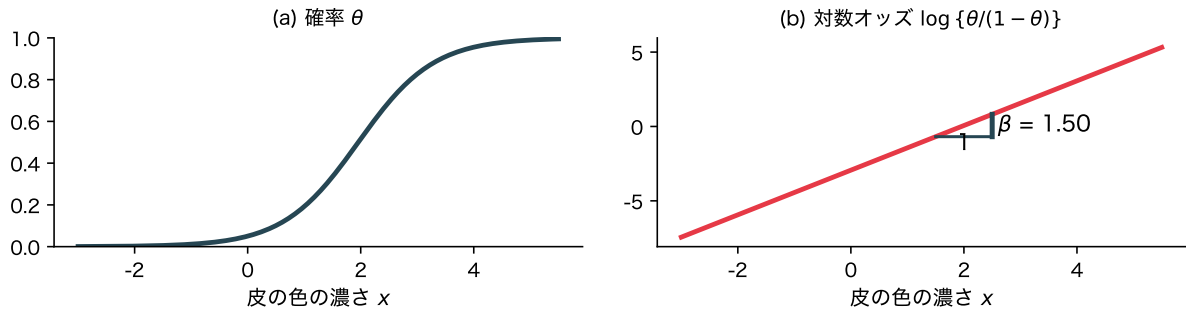
図 11: みかんの人工データに当てたロジスティック回帰。(a) 確率、(b) 対数オッズ。対数オッズは直線で、 x が 1 増えると \hat{\beta} だけ上がる
