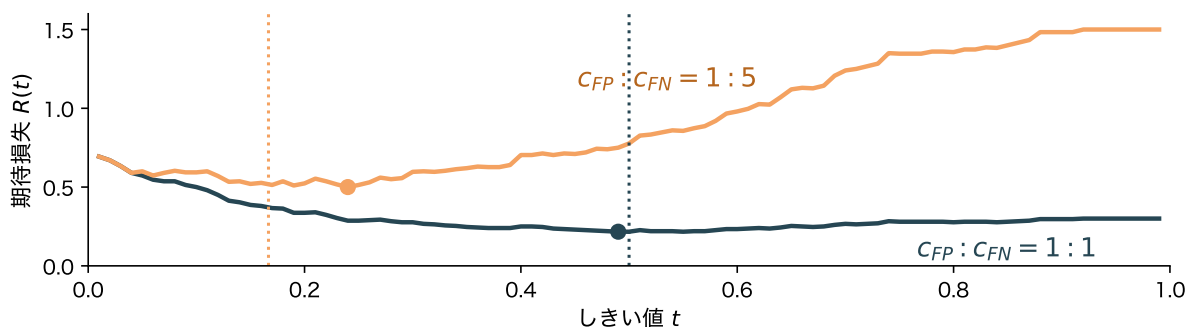
図 13: 与信データのテスト(300 人)で数えた期待損失 R(t) 。点は谷底、点線は (5) 式の t^* (損失の比 1:1 で 0.5、1:5 で 1/6 )
