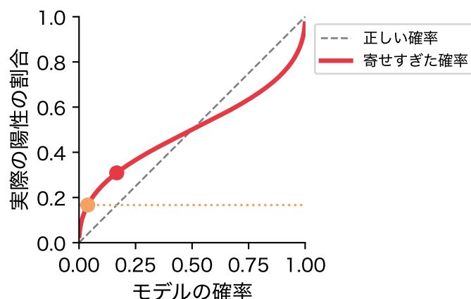
図 11: 較正の概念図。横軸はモデルの確率、縦軸は実際の陽性の割合。破線は較正された確率、赤の曲線は対数オッズを本当の 2 倍に出したモデル
