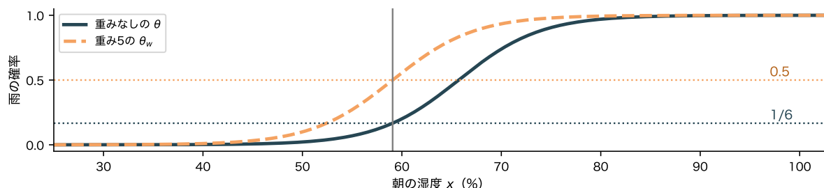
図 10: 雨の日の人工データ(朝の湿度 1 変数)の LDA の事後確率 \theta (実線)と、陽性の行に重み 5 を付けた確率 \theta_w (破線)。 \theta_w = 0.5 と \theta = 1/6 は同じ x (灰の線)で起きる
