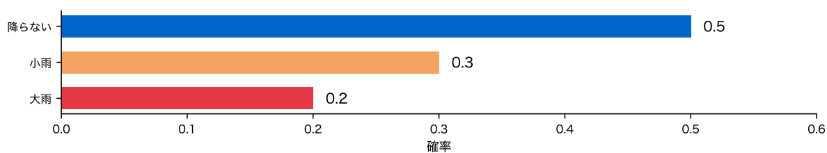
図 2: ある朝の、降らない・小雨・大雨の確率
