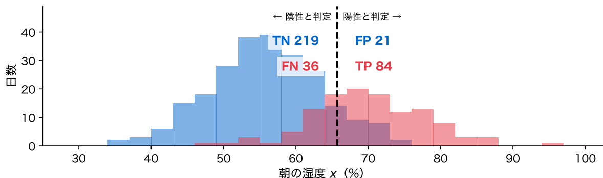
図 3: 人工的な 360 日を朝の湿度で並べ(降らなかった日が青、降った日が赤)、LDA の事後確率 0.5 (破線)で切ったときの 4 つのマスの日数
