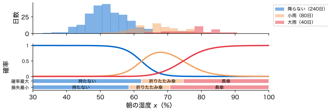
図 8: 降らない・小雨・大雨の人工的な 360 日。上は朝の湿度の分布、下は 3 群の LDA の確率と、湿度ごとに選ぶ支度 (確率最大で選ぶ帯と、表 1 の損失で選ぶ帯)
