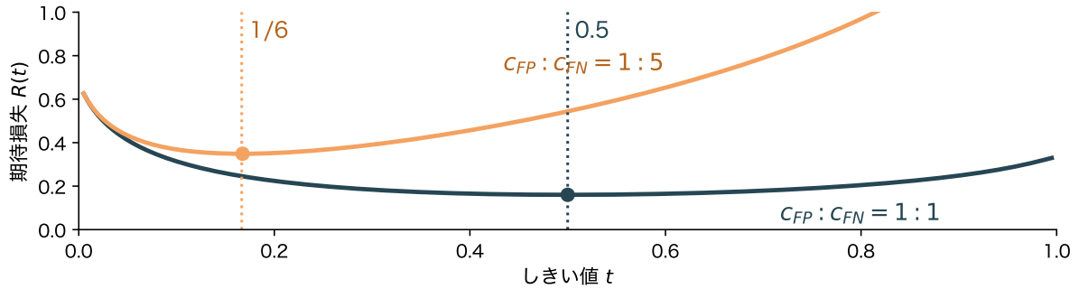
図 4: 雨の日の人工データで推定した正規分布のモデルで計算した期待損失 R(t) 。点は谷底、点線は (5) 式の t^* (損失の比 1:1 で 0.5、1:5 で 1/6)
