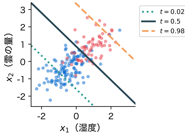
図 9: 朝の湿度と雲の量(標準化)の 2 変数の人工データに LDA を当て、事後確率が 0.02 (点線)・0.5 (実線)・0.98 (破線)になる境界を引いたもの
