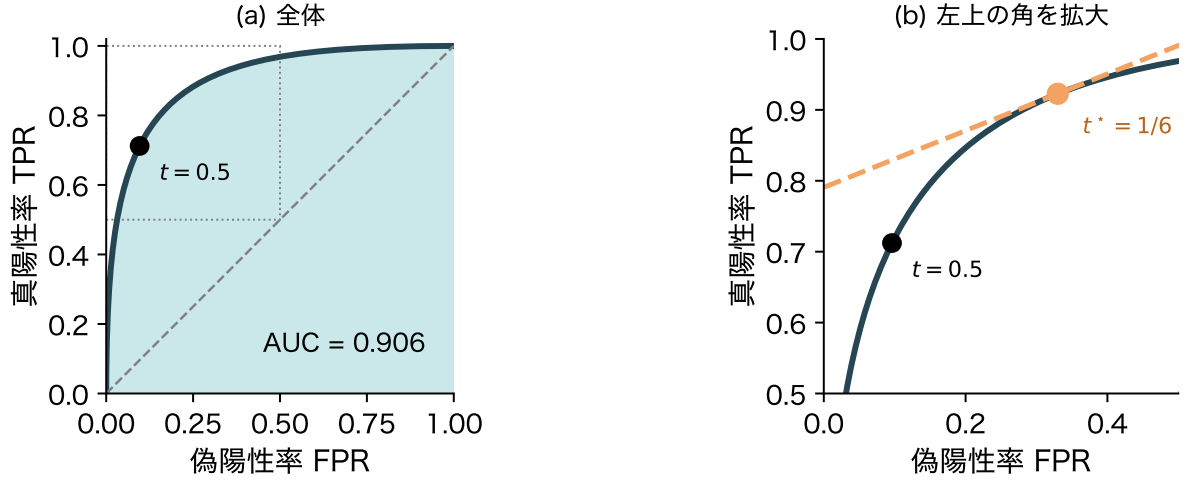
図 6: 雨の日の人工データで推定した正規分布のモデルの ROC 曲線。(a) 全体。色を塗った部分の面積が AUC、黒の点は t = 0.5 。(b) (a) の点線の枠(左上の角)を拡大したもの。橙の点は損失の比 1:5 の t^* = 1/6 、橙の破線は期待損失が R(t^*) に等しい点の直線 (7) 式
