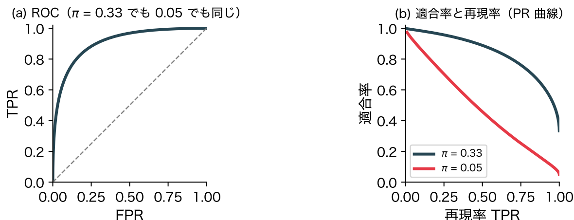
図 7: 図 6 と同じモデルで、陽性の割合 \pi だけを変えたときの (a) ROC 曲線と (b) PR 曲線
