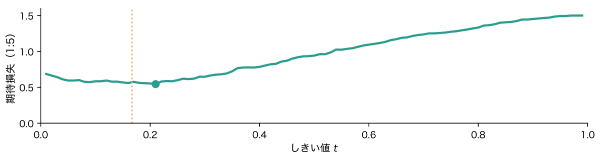
図 16: 与信データの訓練 700 人で、5 分割の交差検証の確率から数えた期待損失(損失の比 1:5)。点は谷底、点線は t^* = 1/6
