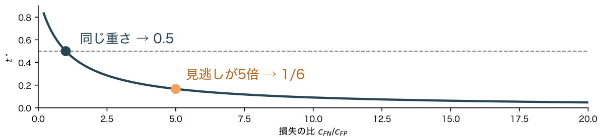
図 5: 損失の比 c_{FN}/c_{FP} と最適なしきい値 t^* = 1/(1 + c_{FN}/c_{FP})
