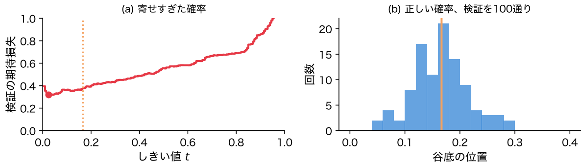
図 12: 検証の行でしきい値を選ぶ。(a) 寄せすぎた確率のモデルで、検証の 1000 日で数えた期待損失(損失の比 1:5)。(b) 確率が正しいモデルで、検証の 360 日を 100 通り作り直したときの谷底の位置
