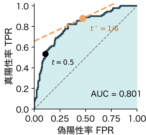
図 15: 与信データのテスト(300 人)での ROC 曲線。色を塗った部分の面積が AUC。黒の点は t = 0.5 、橙の点は t^* = 1/6 、橙の破線は損失の比 1:5 の等損失線
