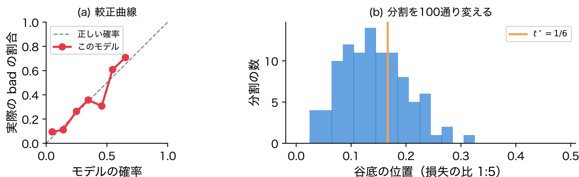
図 14: 与信データの谷底のずれの出どころ。(a) テストの確率の較正曲線(20 人以上の区間)。(b) 分割を 100 通り変えたときの、損失の比 1:5 の谷底の位置
