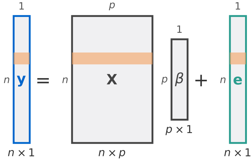
図 7: 重回帰のモデル y = X\beta + e を四角形で描いたもの(概念図)。箱の縦は行の数、横は列の数。帯は第 i 行
