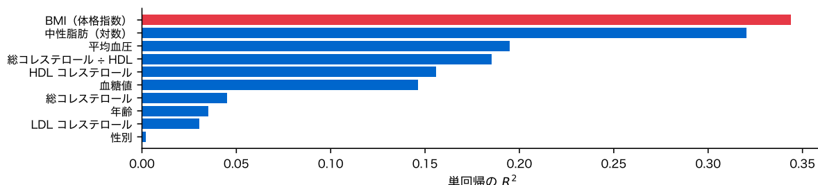
図 10: 説明変数を 1 つずつ使った単回帰の決定係数
