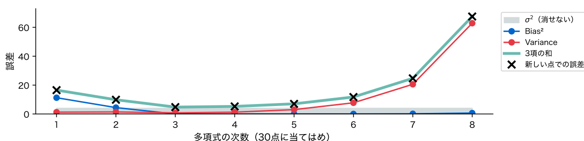
図 7: 人工データでのバイアス・バリアンス分解。30 点の訓練データを 300 回取り直して計算した 3 項と、その和(緑)、新しい点で直接測った誤差(X)
