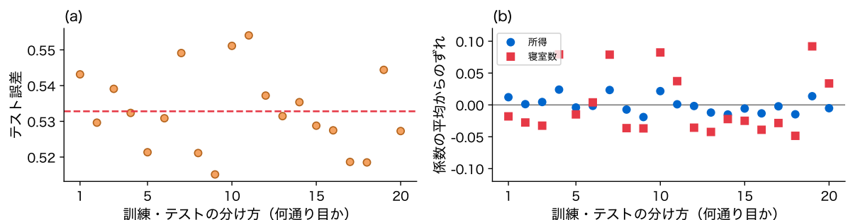
図1: カリフォルニアの住宅価格の8列のモデルを、訓練・テストへの分け方だけを20回当てはめ直した結果。(a) テスト誤差、(b) 所得(青)と寝室数(赤)の係数(標準偏差1つぶんあたり)の、20通りの平均からのずれ
