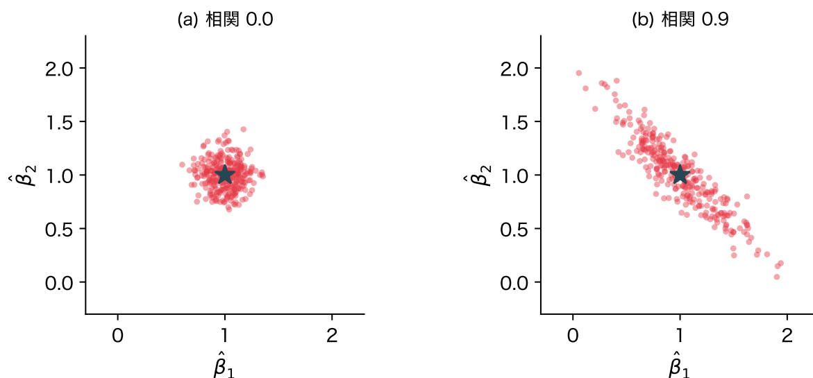
図 6: 人工データで y を 300 回取り直したときの係数の推定値。★は真の値。(a) 2 列の相関が 0、(b) 0.9
