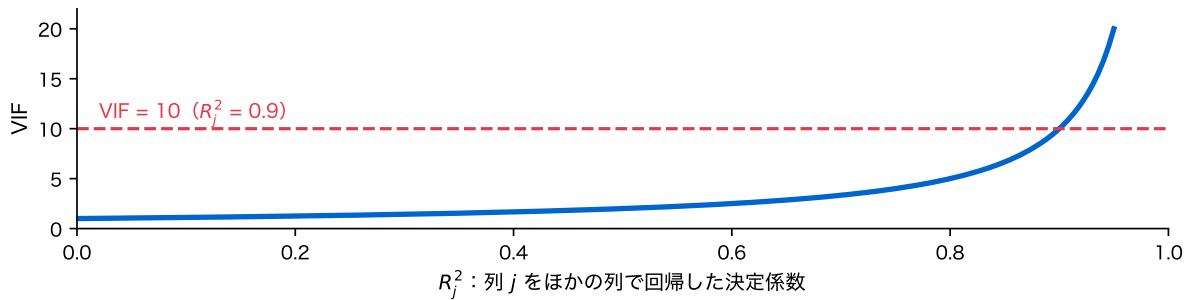
図 7: 分散拡大係数 VIF_j = 1/(1 - R_j^2) と、目安とされる VIF = 10 (赤の破線)
