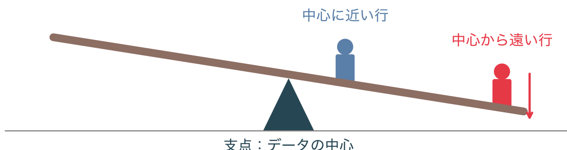
図 10: てこ比のたとえ(概念図)。直線はデータの中心を支点に回る板で、中心から遠い行ほど板を大きく傾ける
