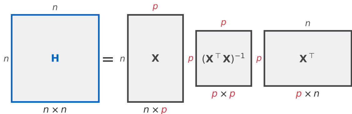
図 8: 射影行列 \mathbf{H} = \mathbf{X}(\mathbf{X}^\top \mathbf{X})^{-1} \mathbf{X}^\top の大きさ(概念図)。箱の縦は行の数、横は列の数。赤は掛け算でそろった次元
