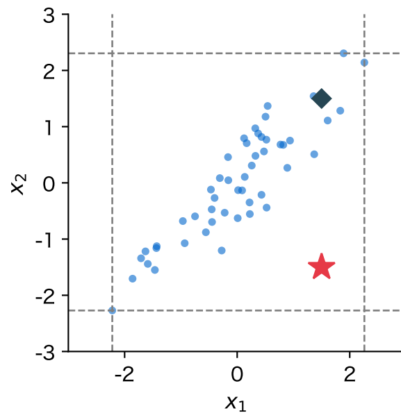
図 13: 相関 0.9 の 2 列(人工データ、50 行)。破線は各列の最小値と最大値。★はどちらの列も範囲の中だが雲の外点、◆は原点から同じ遠さで雲に沿った点
