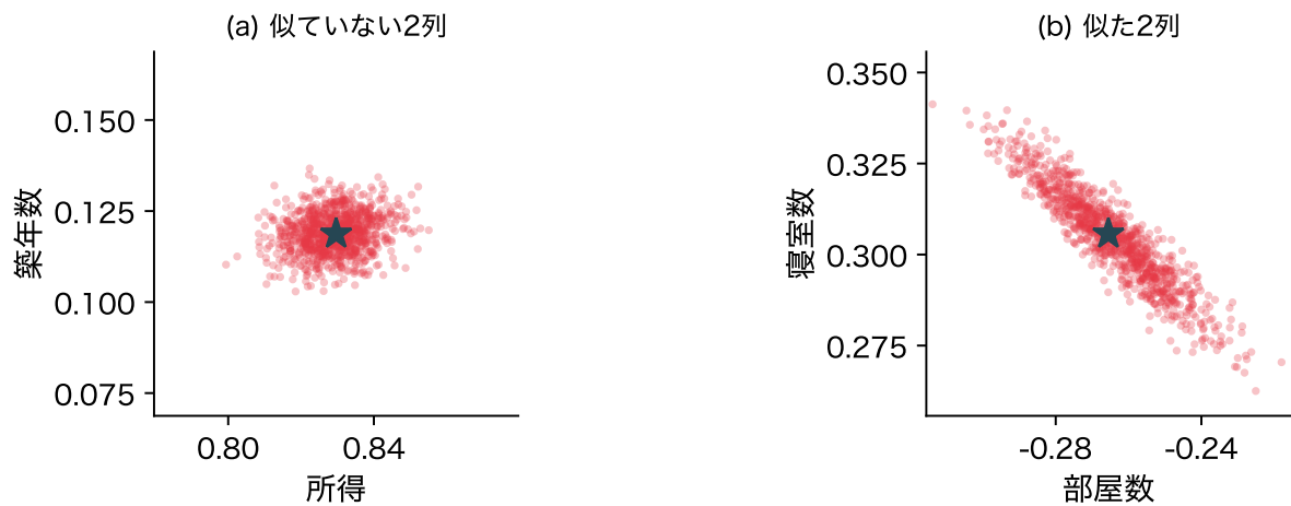
図 18: \mathbf{X} を固定して目的変数を 1000 回作り直したときの係数(標準偏差 1 つぶんあたり)。★は全地区で当てはめた値で、2 枚とも★から \pm 0.05 の範囲を描いた。(a) 所得と築年数、(b) 部屋数と寝室数
