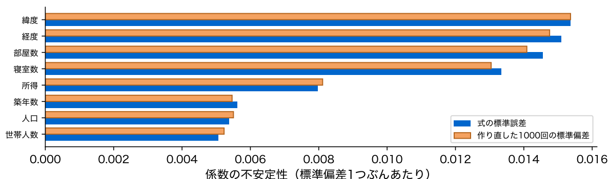
図 17: 係数の不安定性。式 \hat{\sigma}^2(\mathbf{X}^T \mathbf{X})^{-1} による標準誤差(青)と、 \mathbf{X} を固定して目的変数を 1000 回作り直したときの標準偏差(橙)。標準偏差 1 つぶんあたりに直してある
