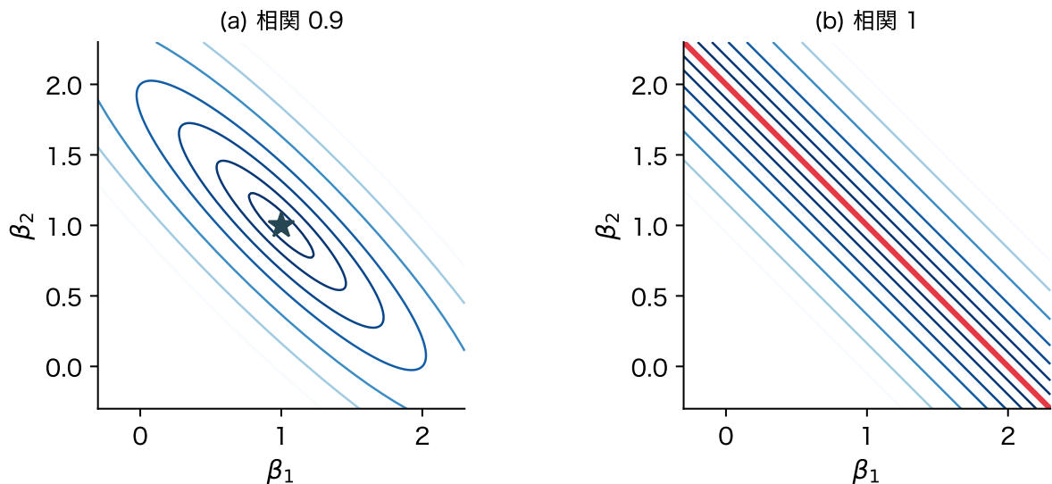
図 14: 2 列の場合の目的関数の等高線(人工データ)。(a) 相関 0.9 では底が 1 点(★)、(b) 相関 1 では底が直線(赤)になり、解が無数にある
