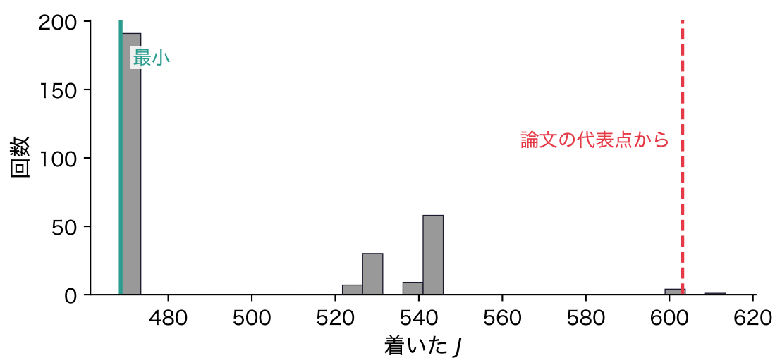
図 9: 100 個体の人工データ、 k = 3 。初期値を変えて着いた J の分布。緑の線が最小、赤の破線が博士論文抜粋の代表点から着いた値
